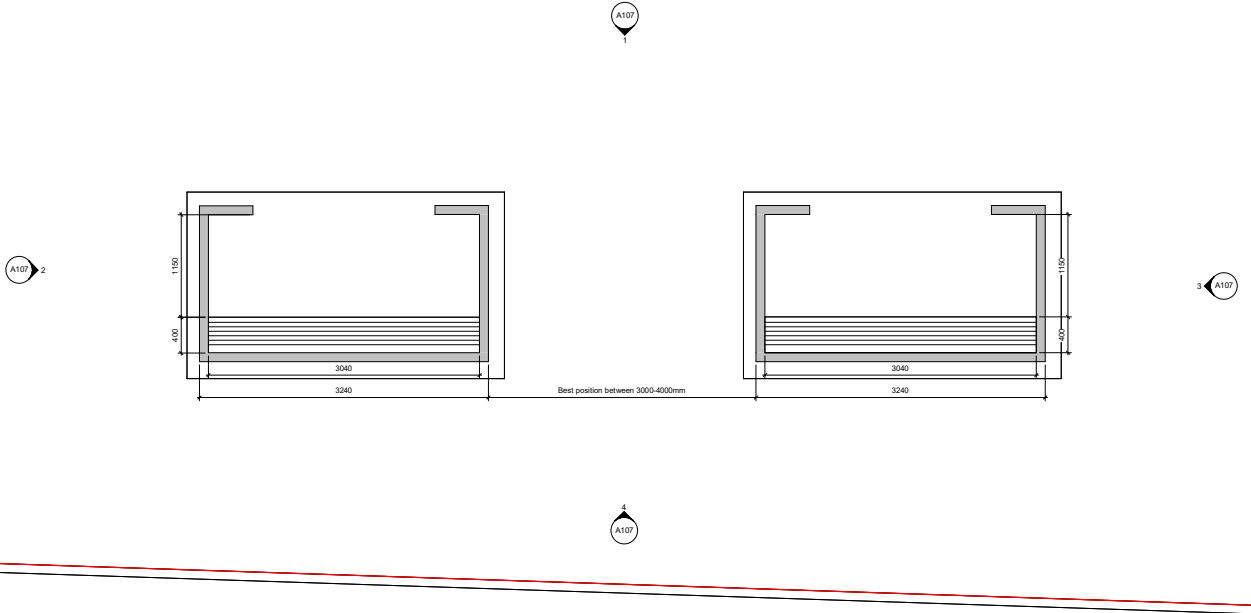
Dugouts Plan 1 : 25
