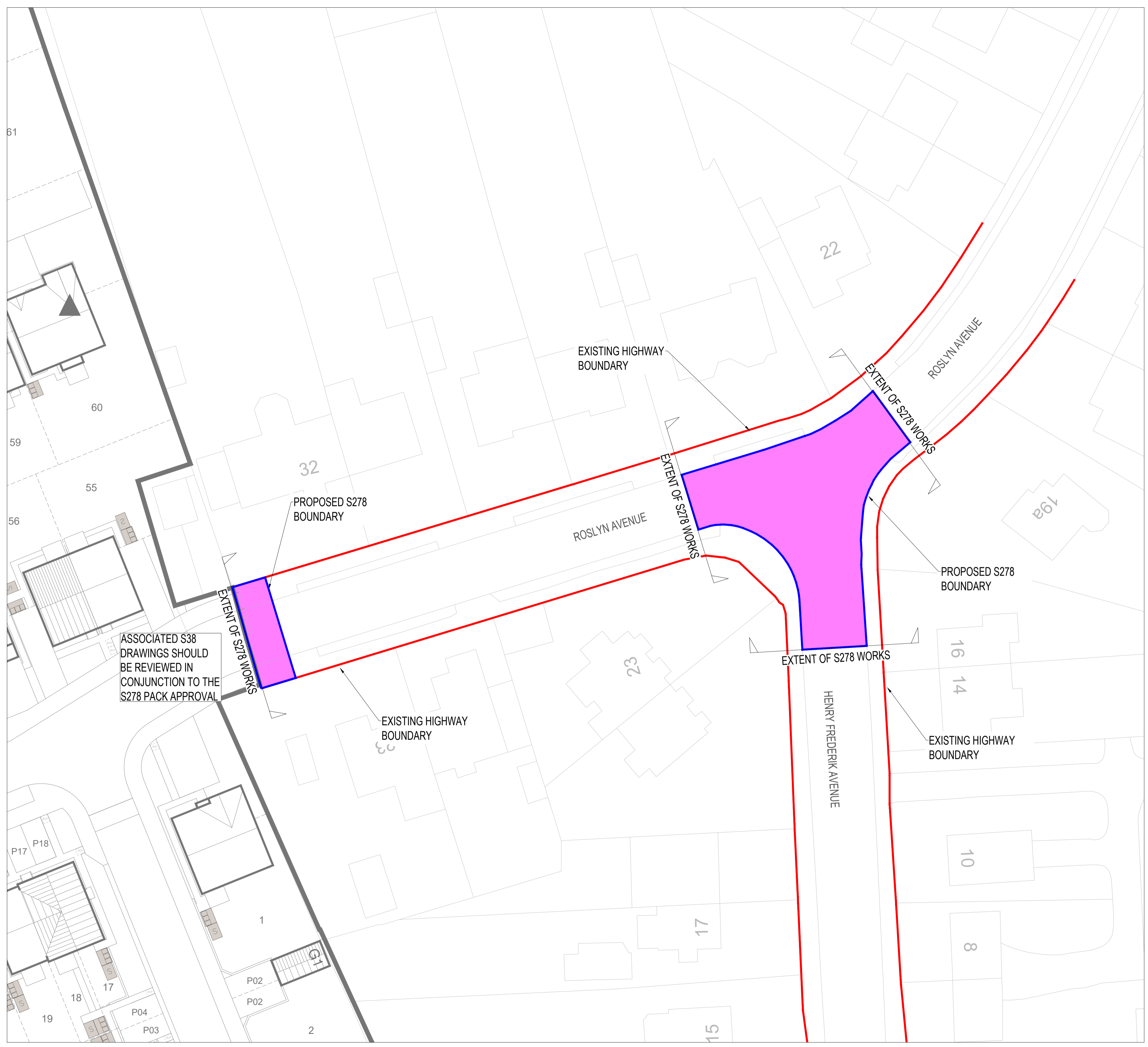
SITE PLAN 1:250
