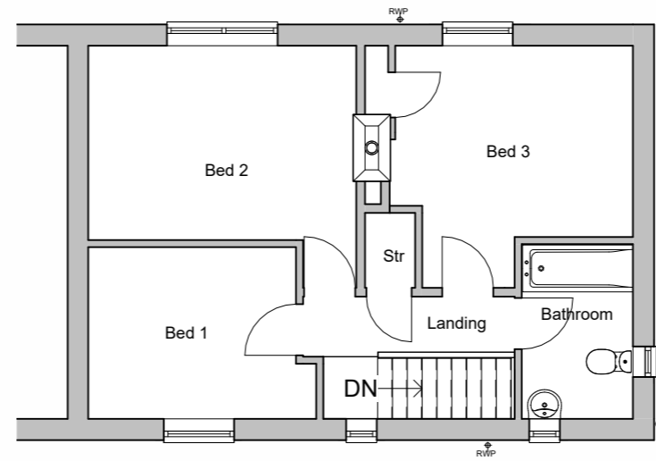
3 03a FF Existing 1 : 100
