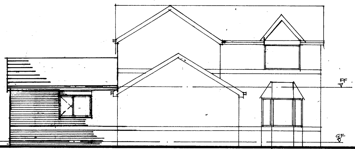
SIDE 1:100
