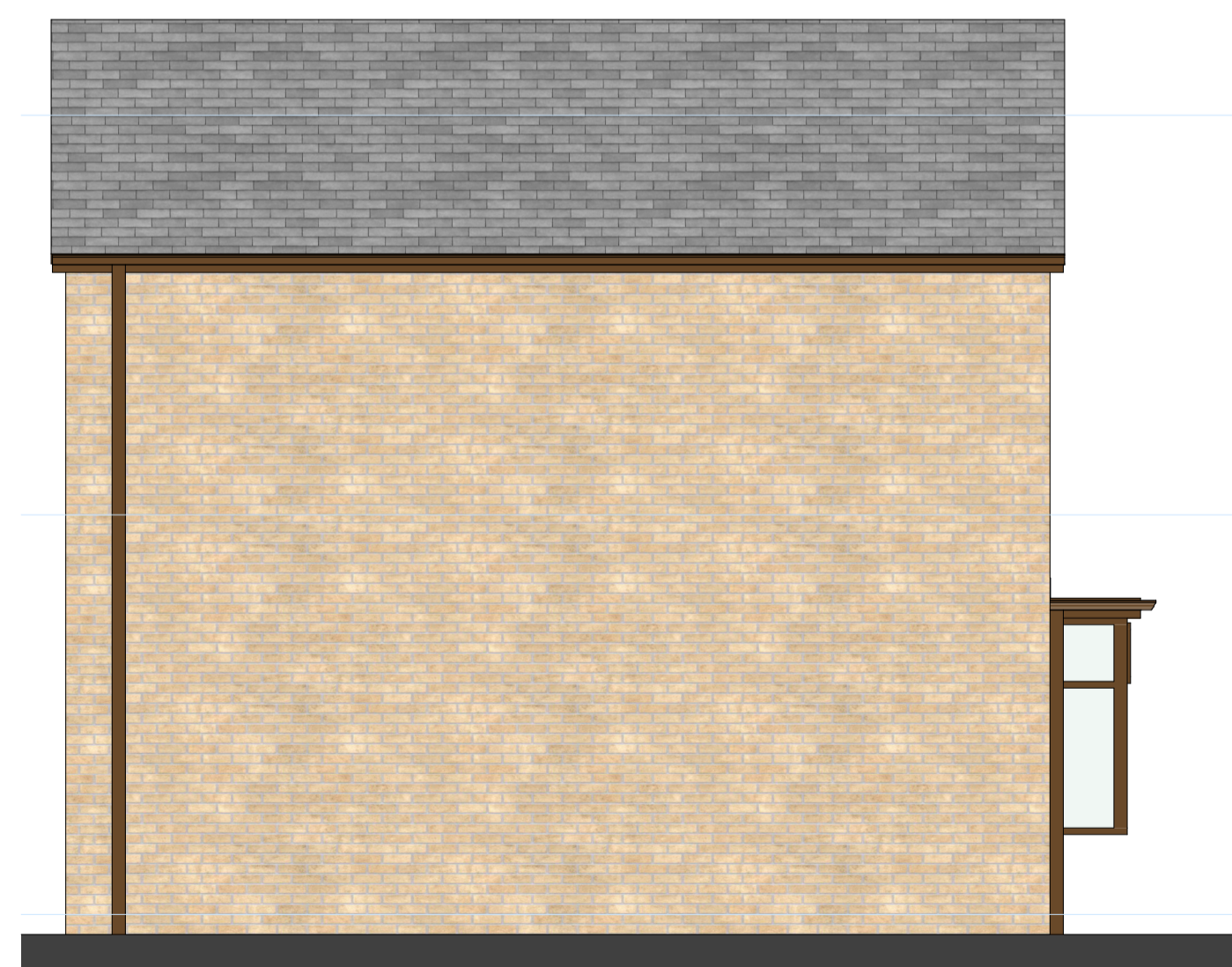
E-04 Elevation 1:50
