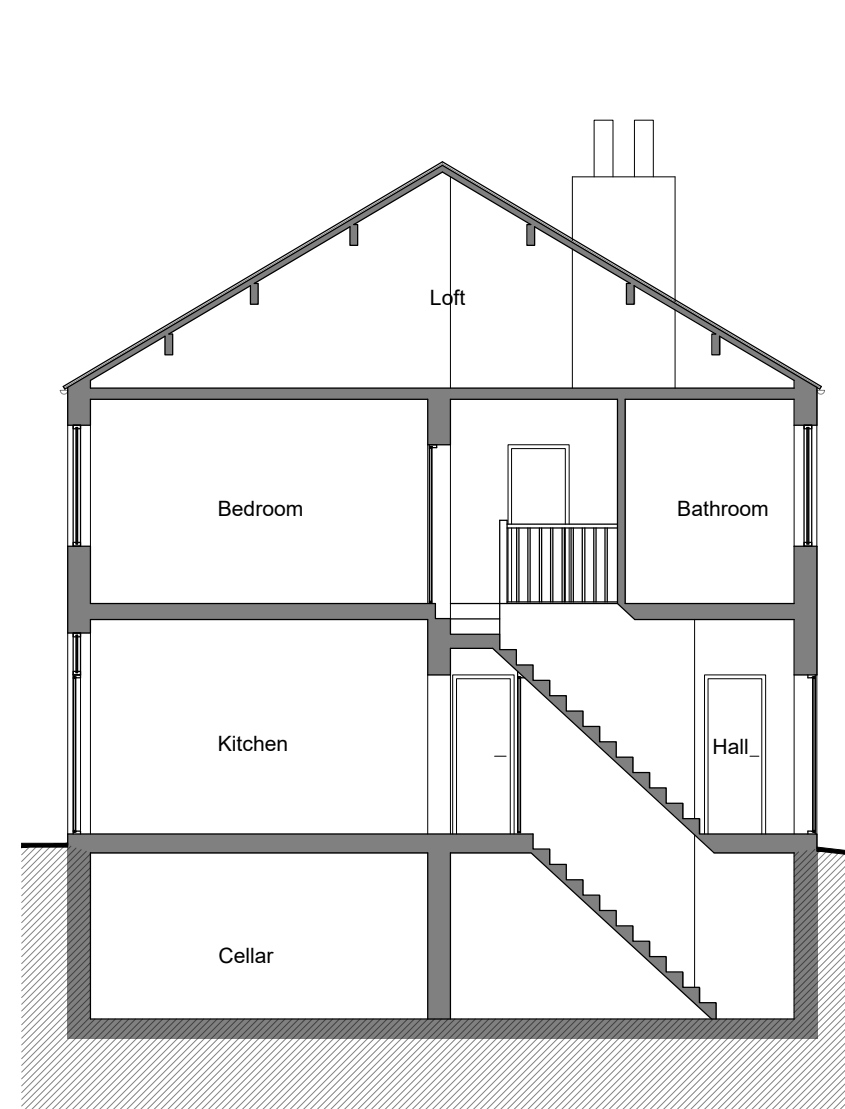
Section A-A : Existing
