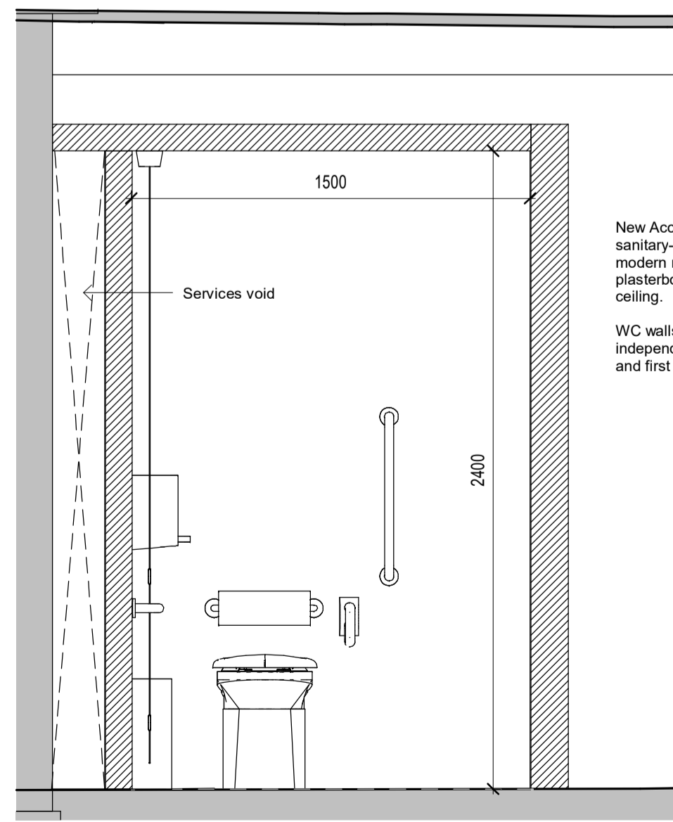
2 Indicative Accessible WC Section 1 : 20
