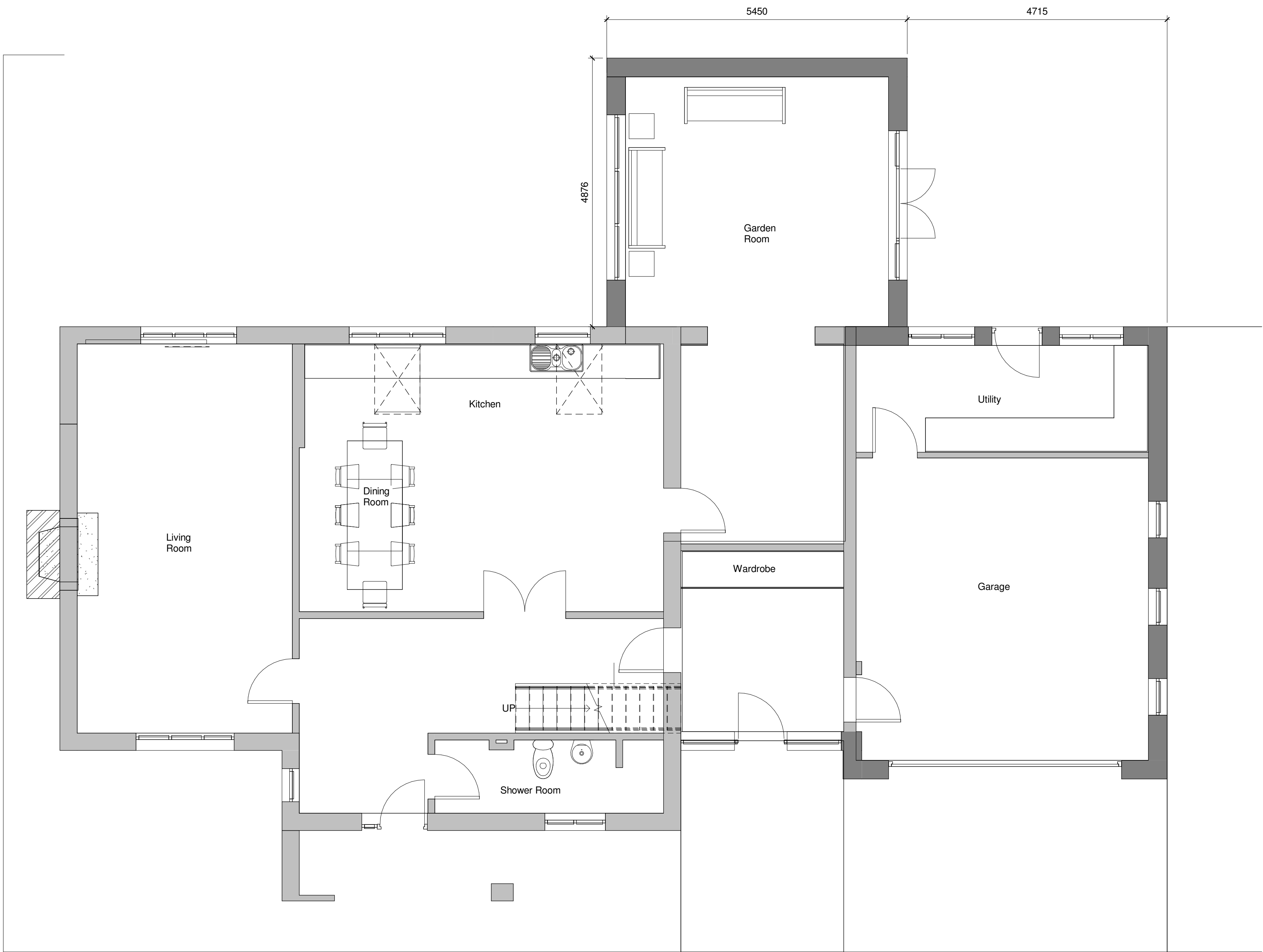
1 Level 0 1 : 50
