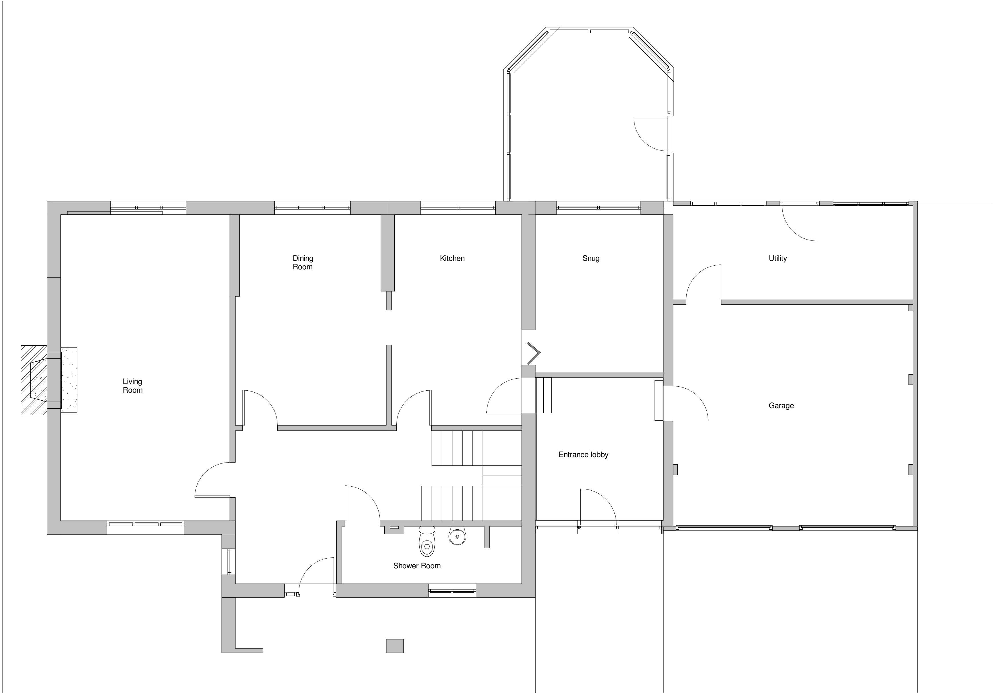
1 Level 0 1 : 50
