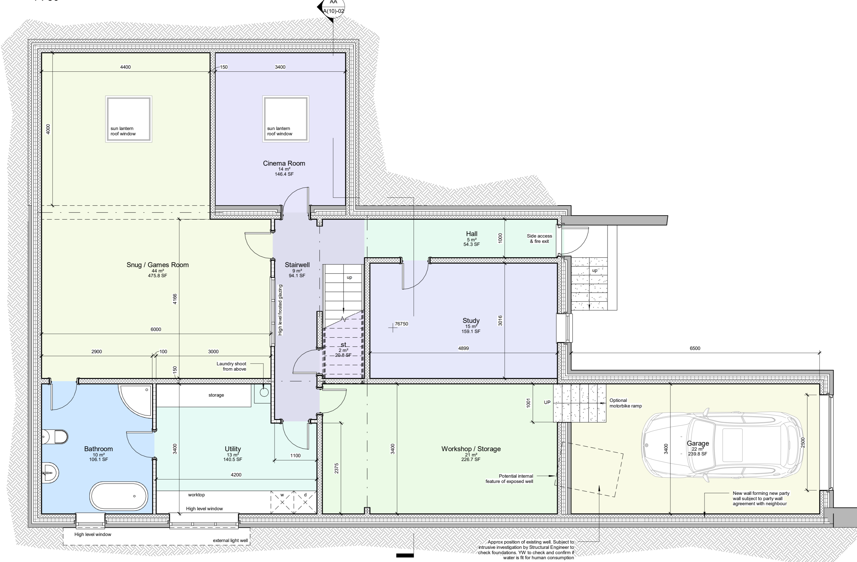
Basement 1 : 50
