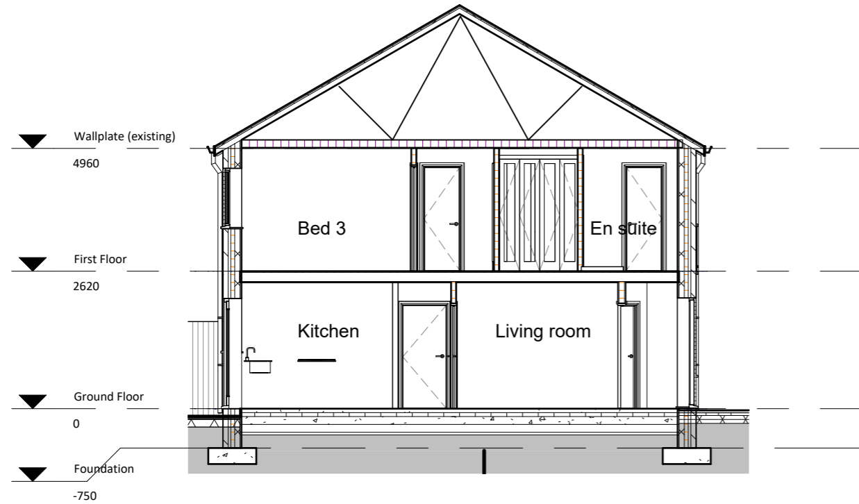
3 Existing Section 1 : 100
