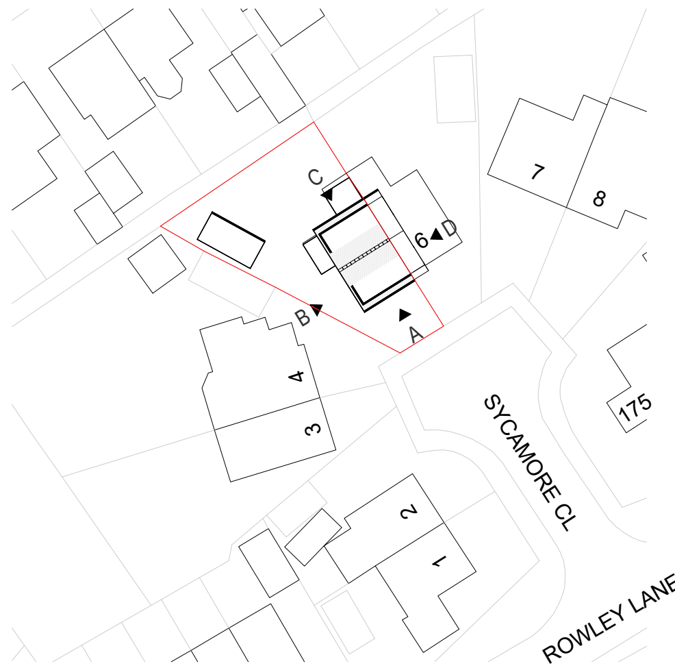
Key Plan 1 : 500
