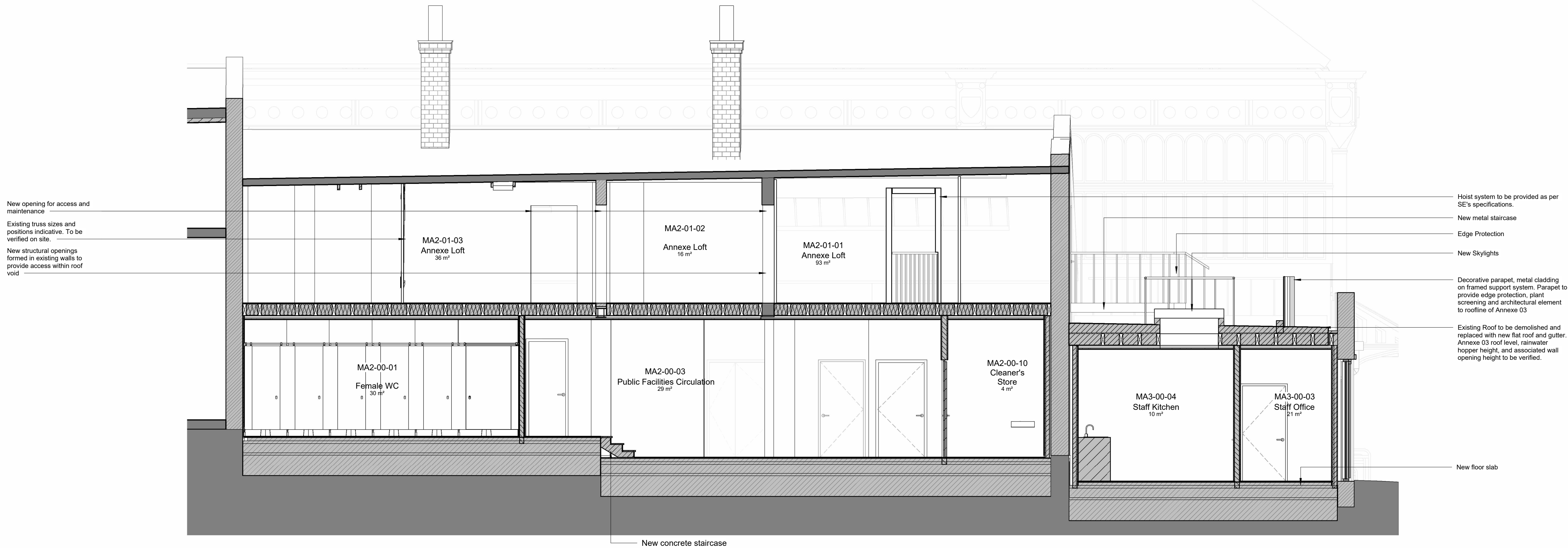
2 Annexe 01 (ER1) and 02 (ER2) - Section 1 : 50
