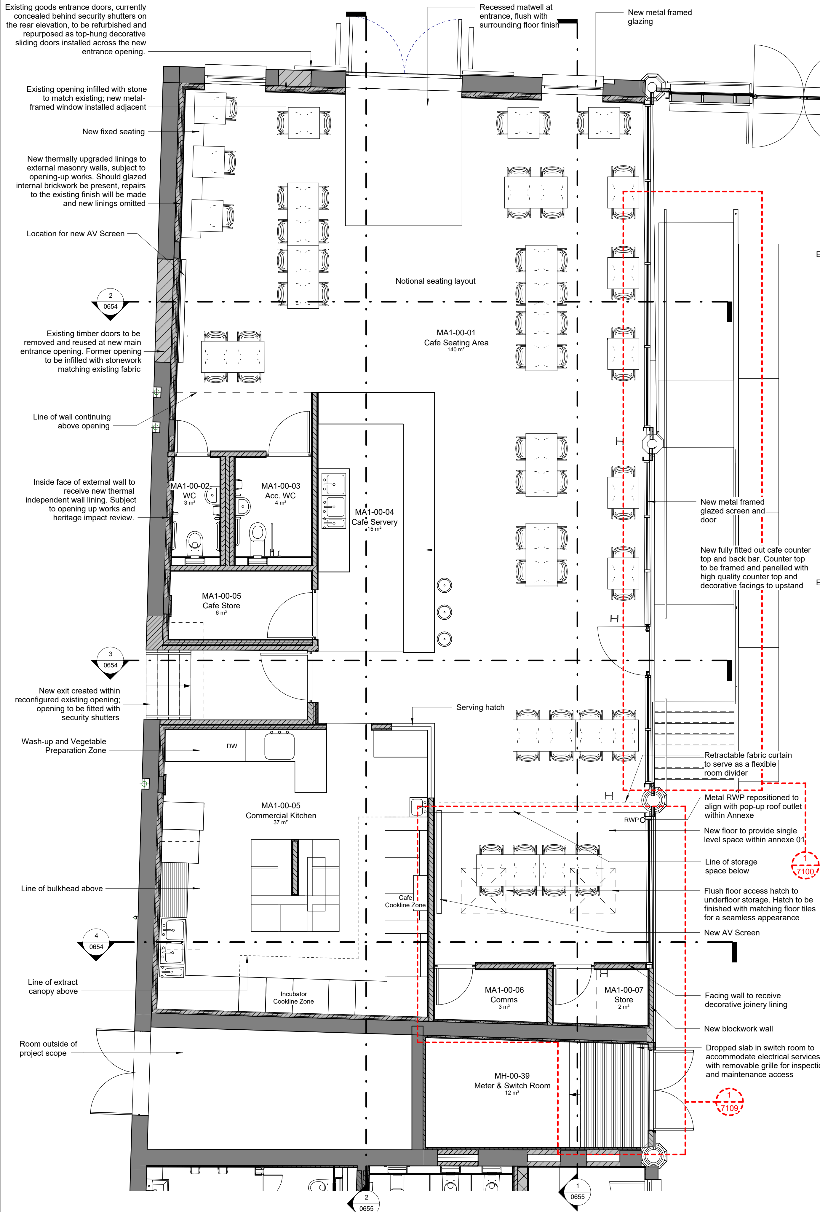
1 Annexe 01 (ER1) - Plan Level 00 1 : 50
