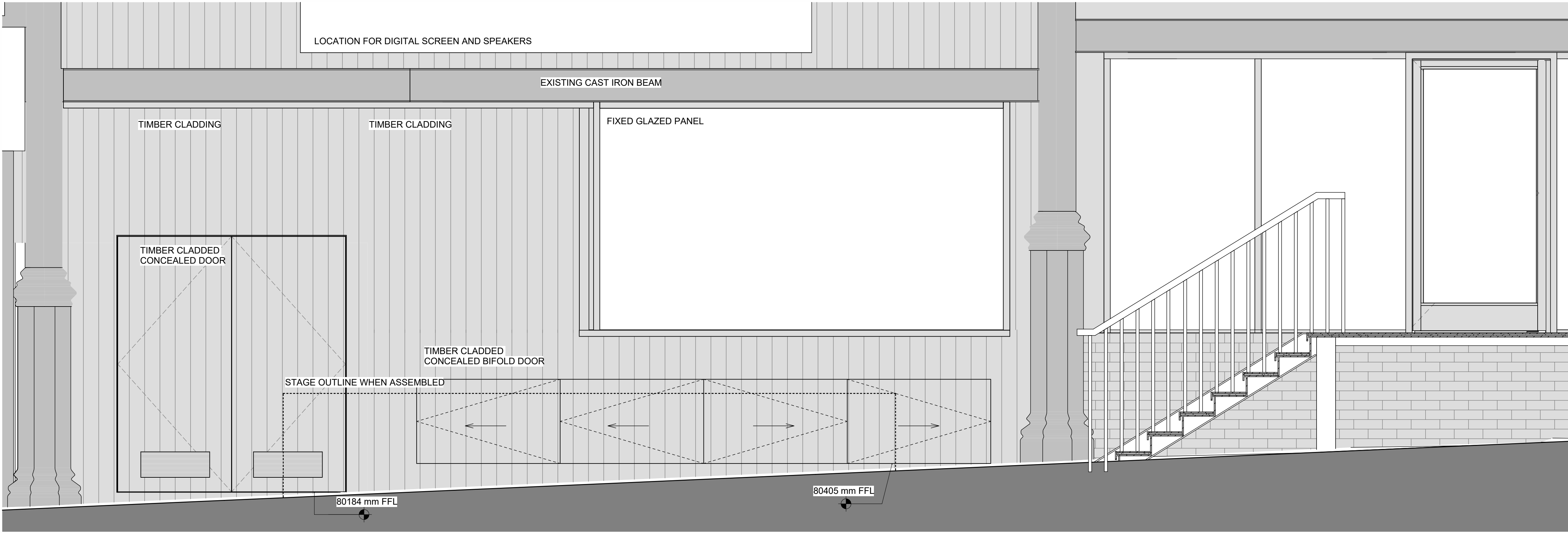
2 Elevation 1 : 20
