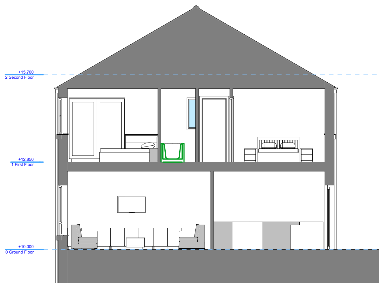
HT F1 Building Section 1:75
