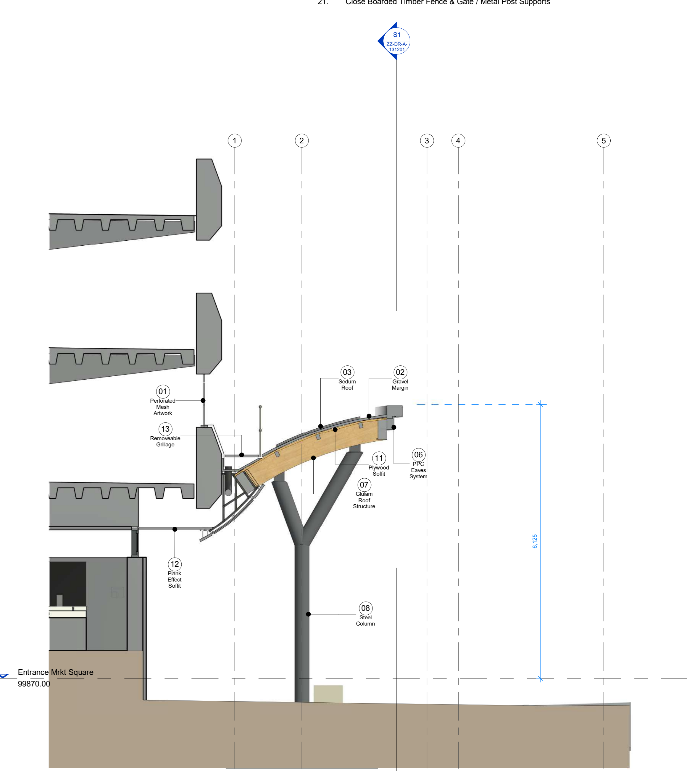
S4 Section 4 Scale: 1 : 50
