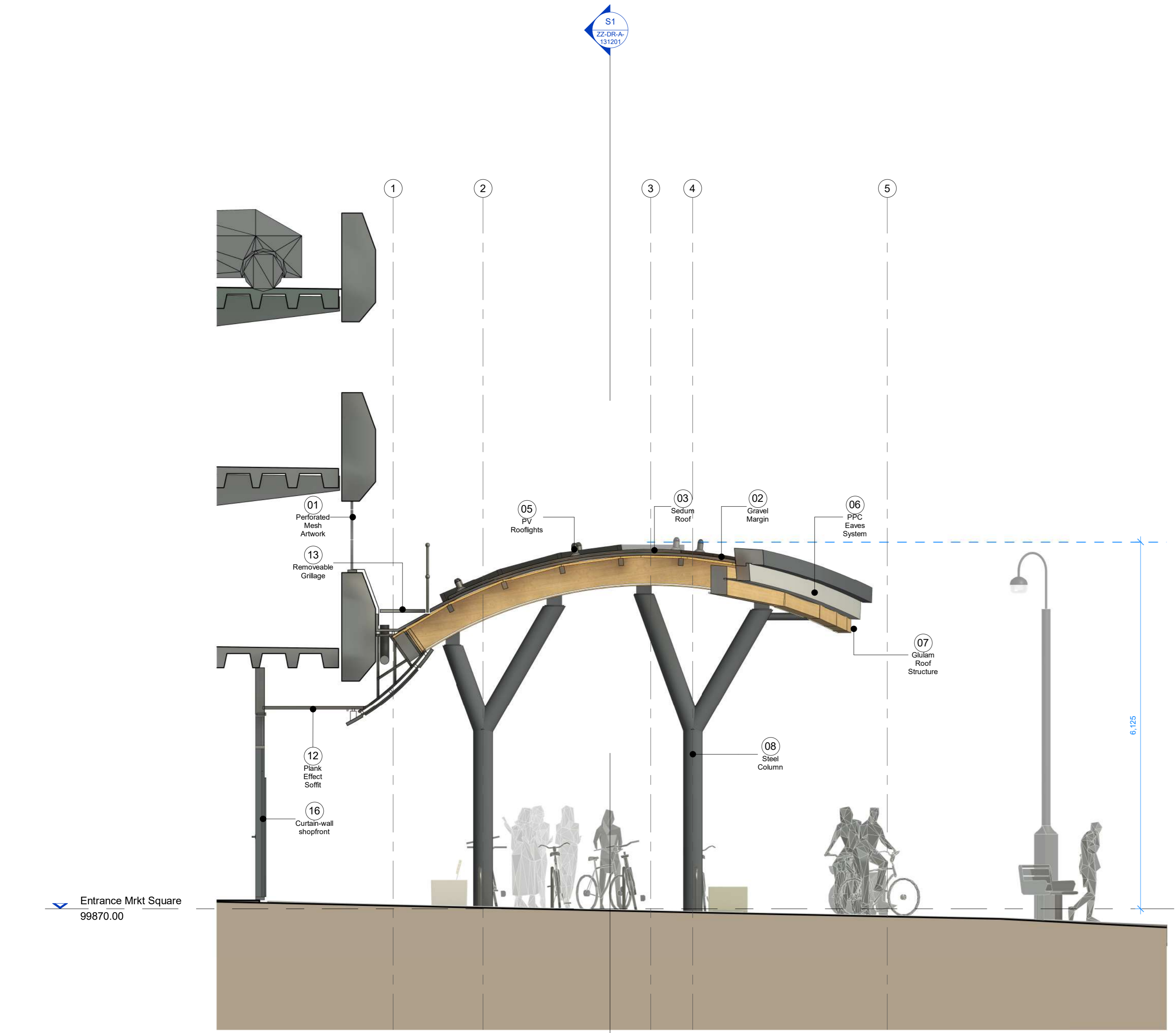
S2 Section 2 Scale: 1 : 50
