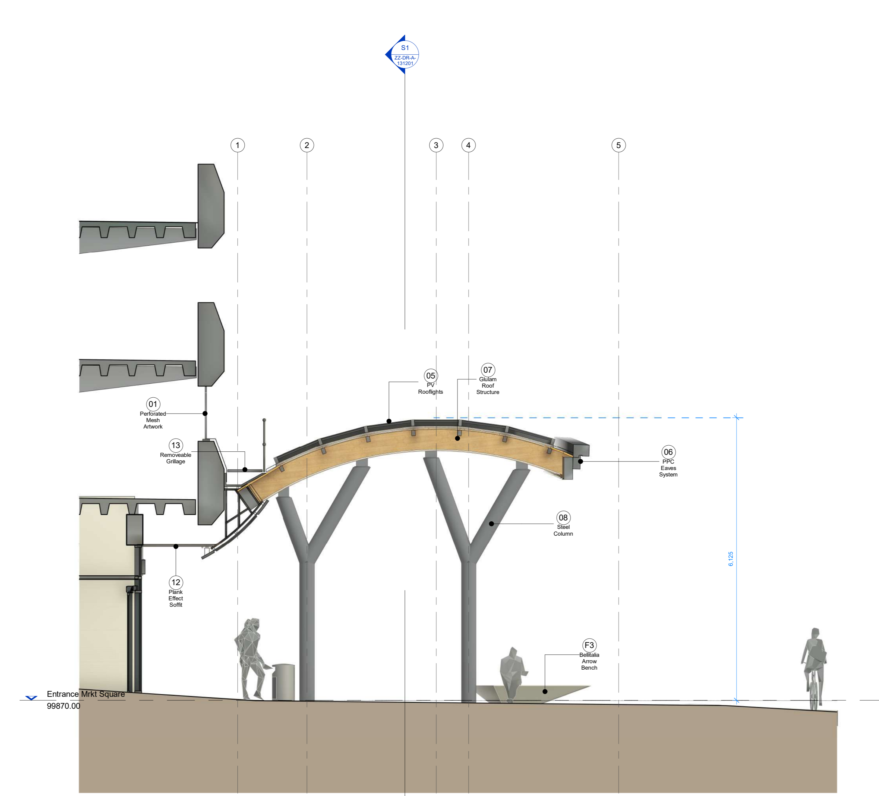
S3 Section 3 Scale: 1 : 50
