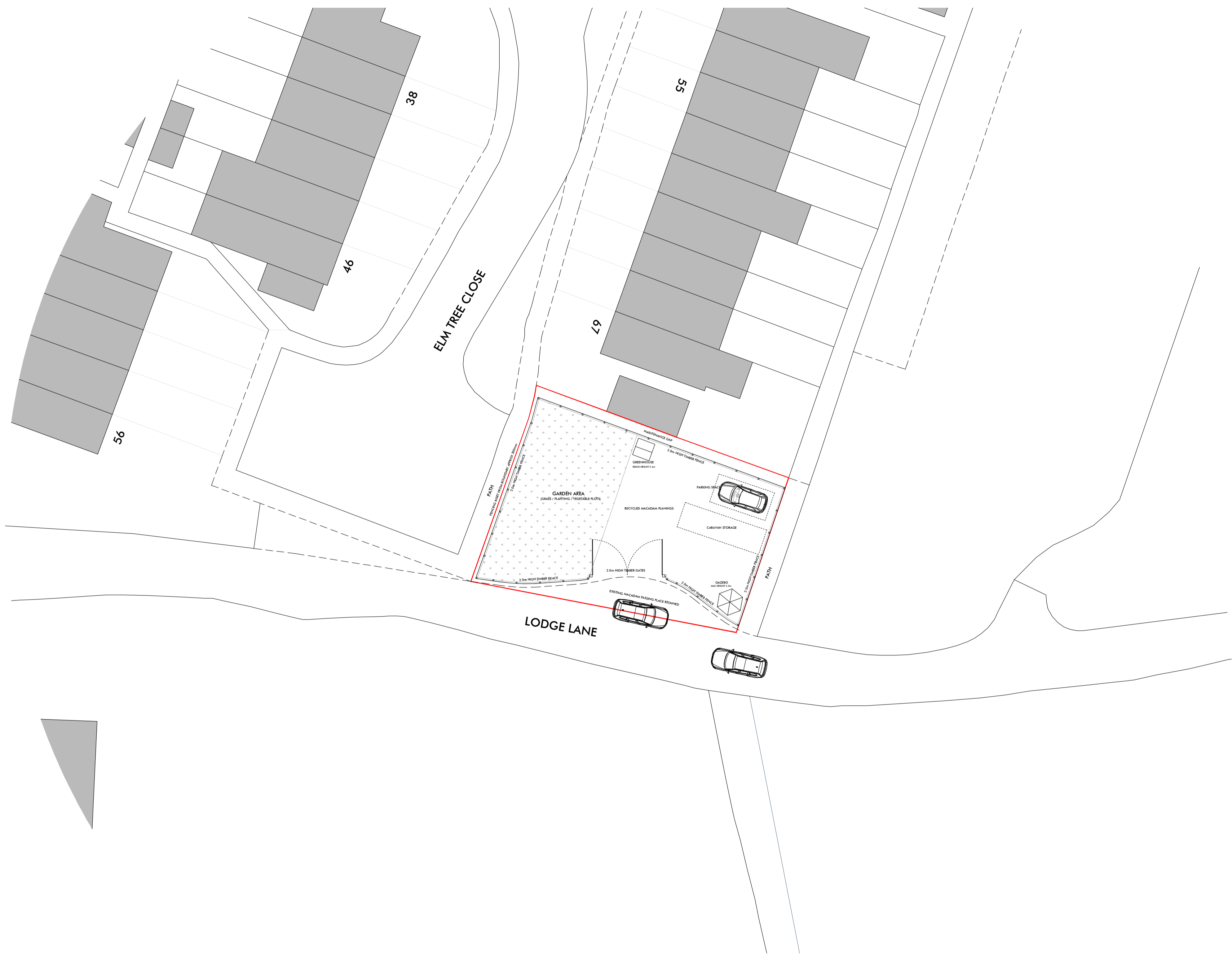
SITE PLAN 1:200
