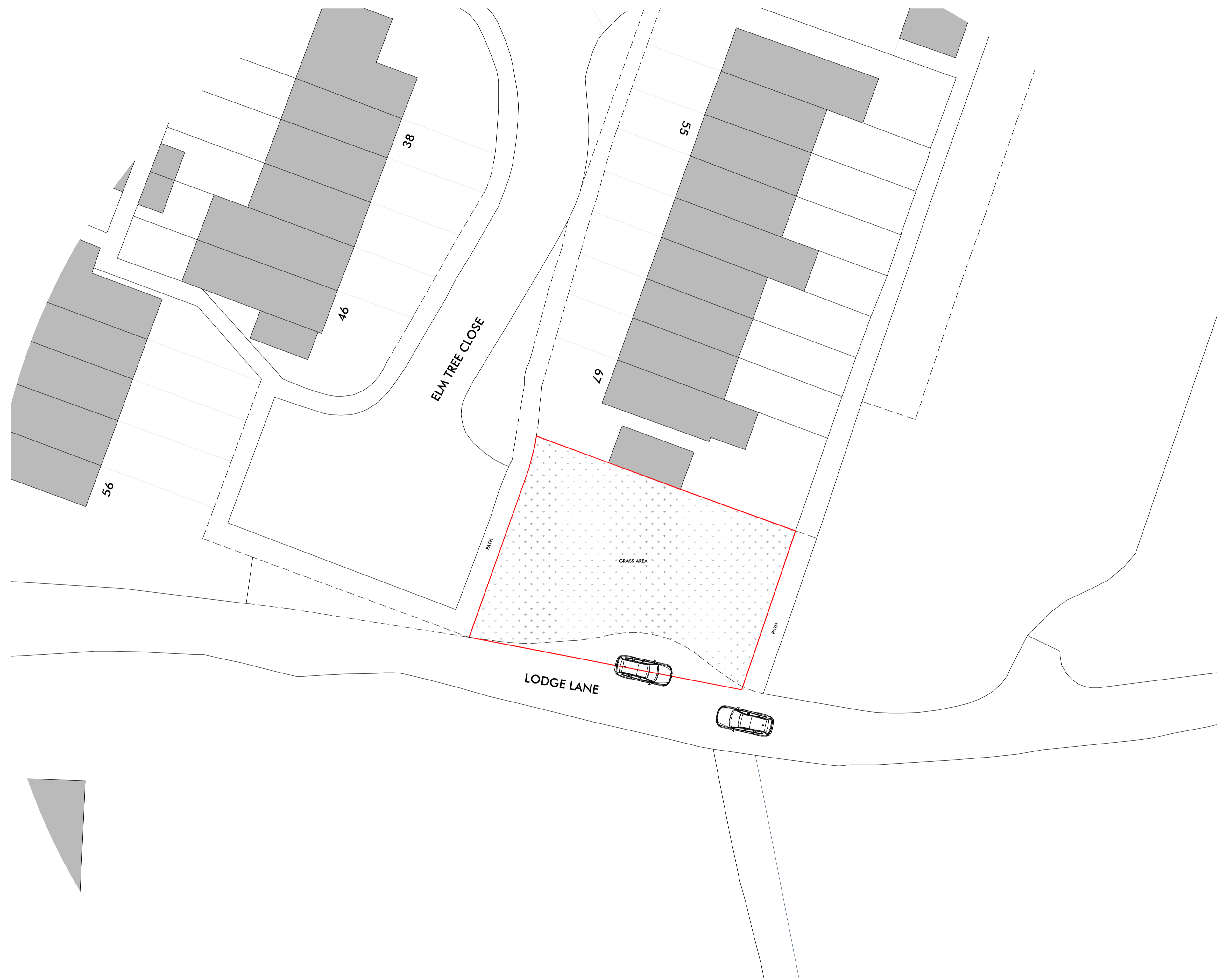
SITE PLAN 1:200
