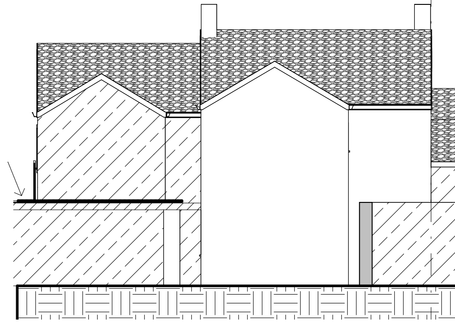
2 South 1 : 100
