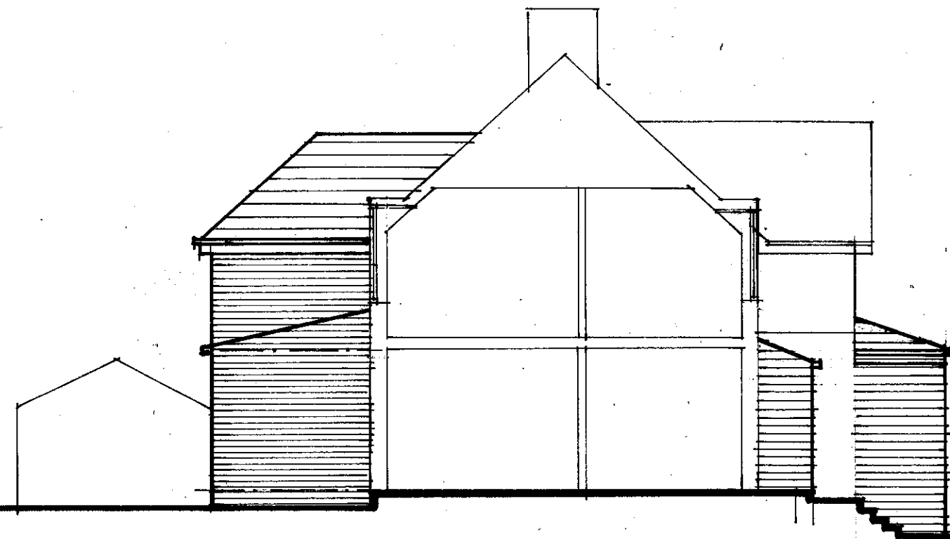
SIDE 1:100
