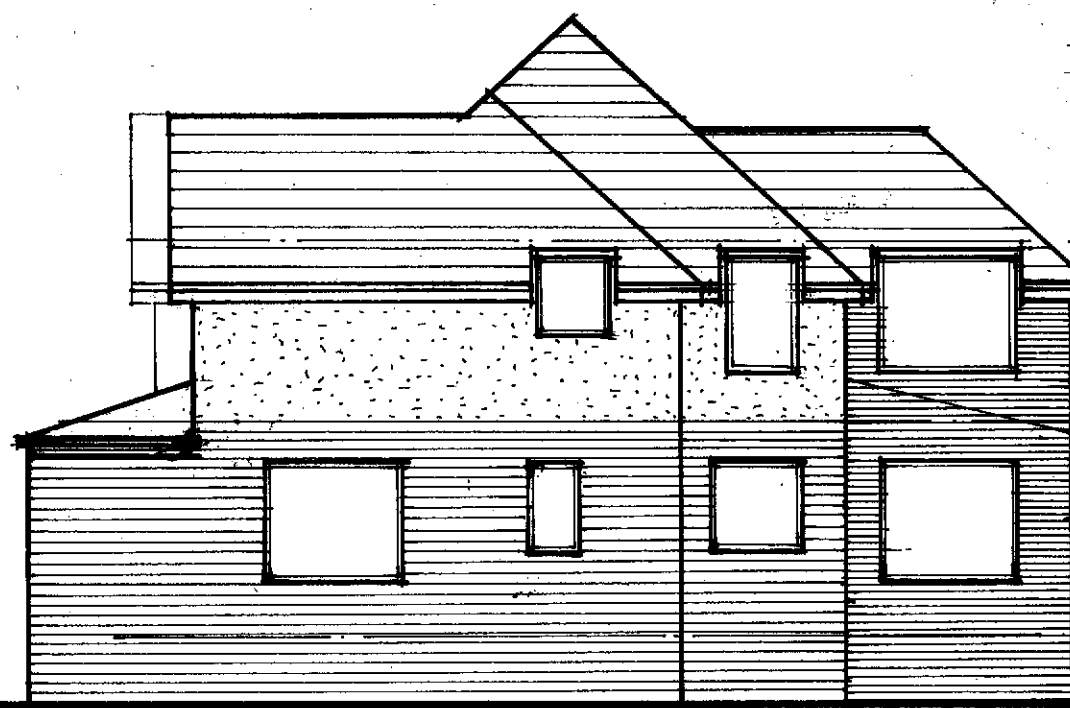
SIDE 1:100
