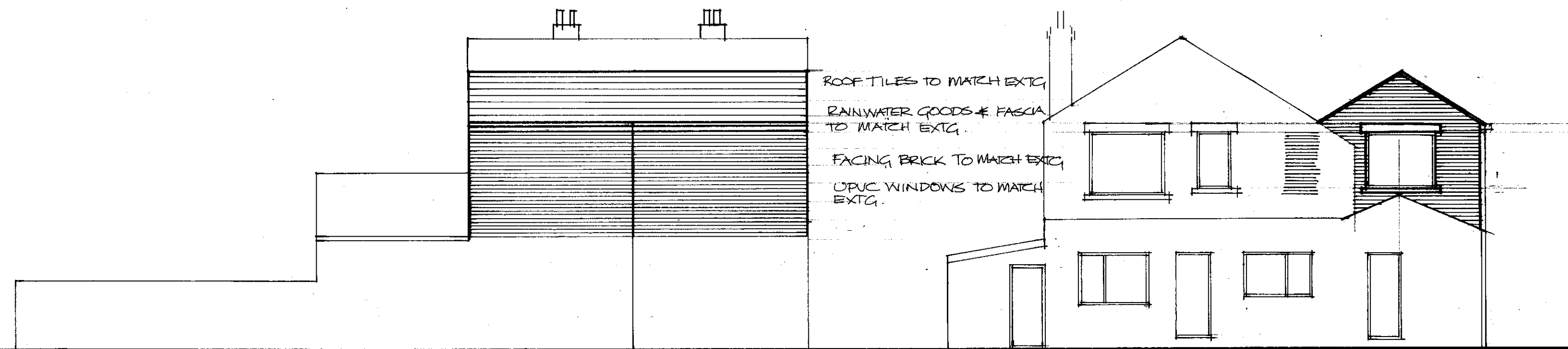
SIDE 1:100
