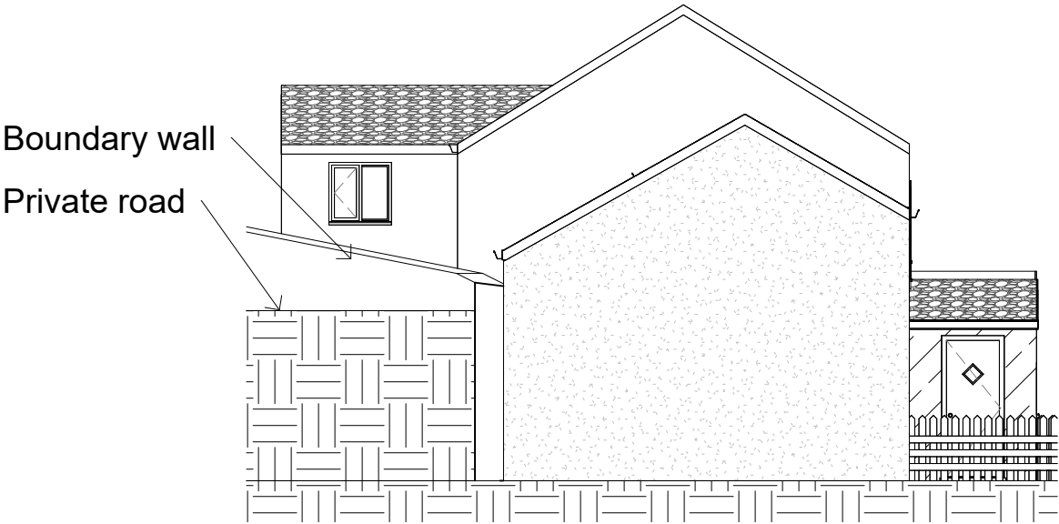
1 North 1 : 100
