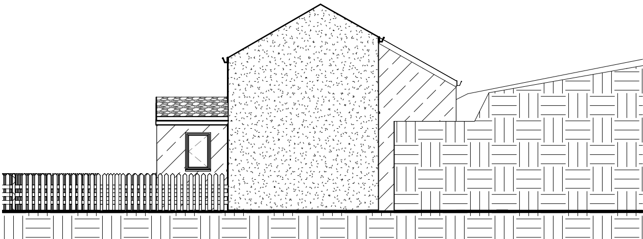
2 South 1 : 100
