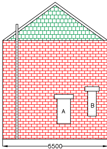
End Elevation
