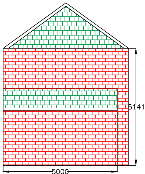
End Elevation
