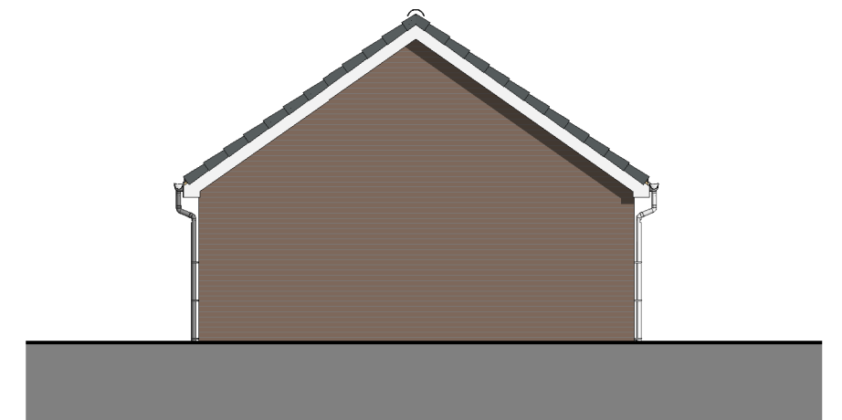
RIGHT ELEVATION
