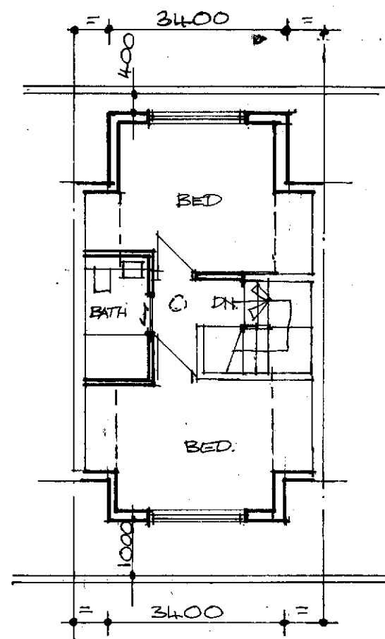
LOFT 1:100
