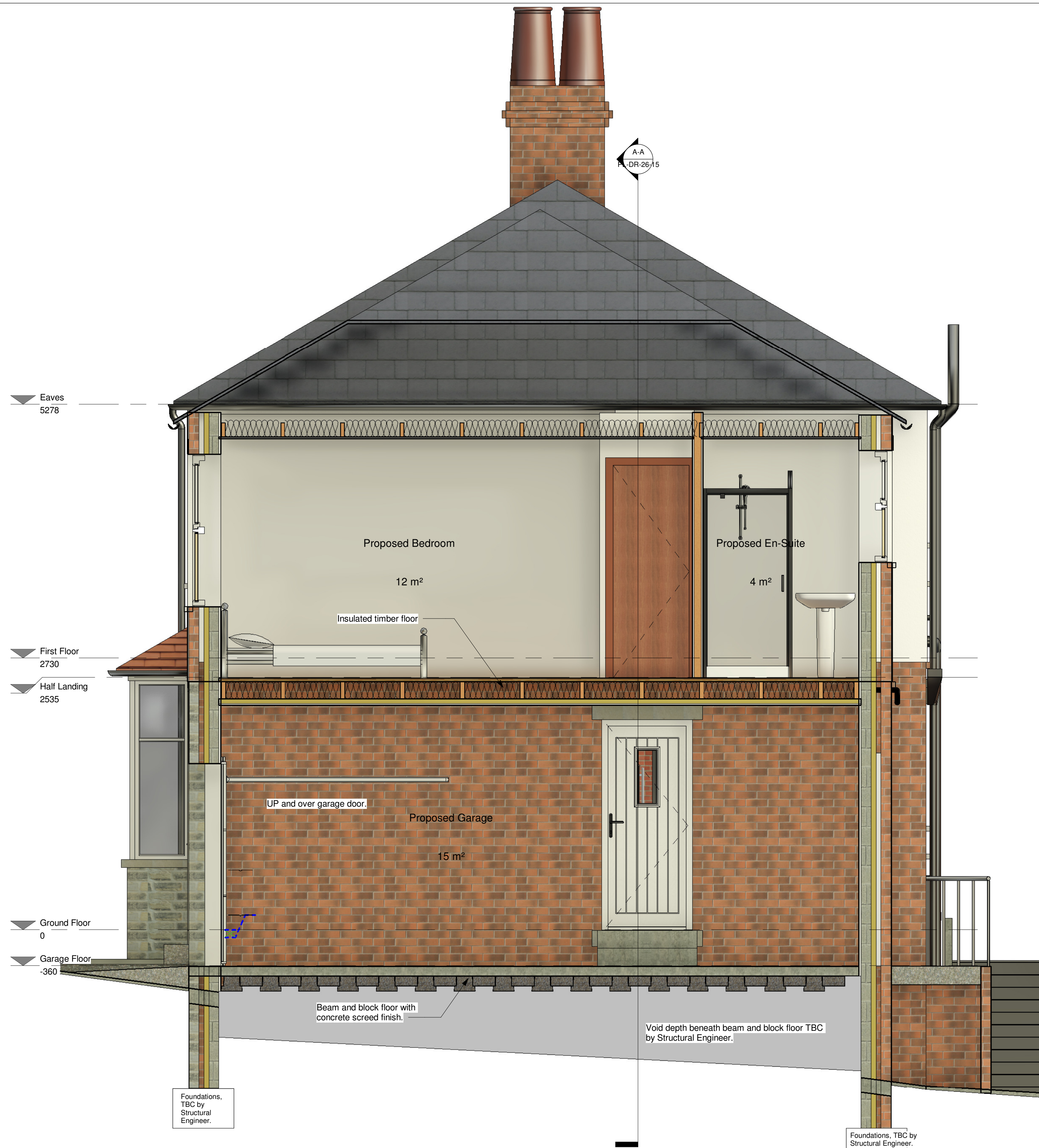
Section B-B 1 : 25
