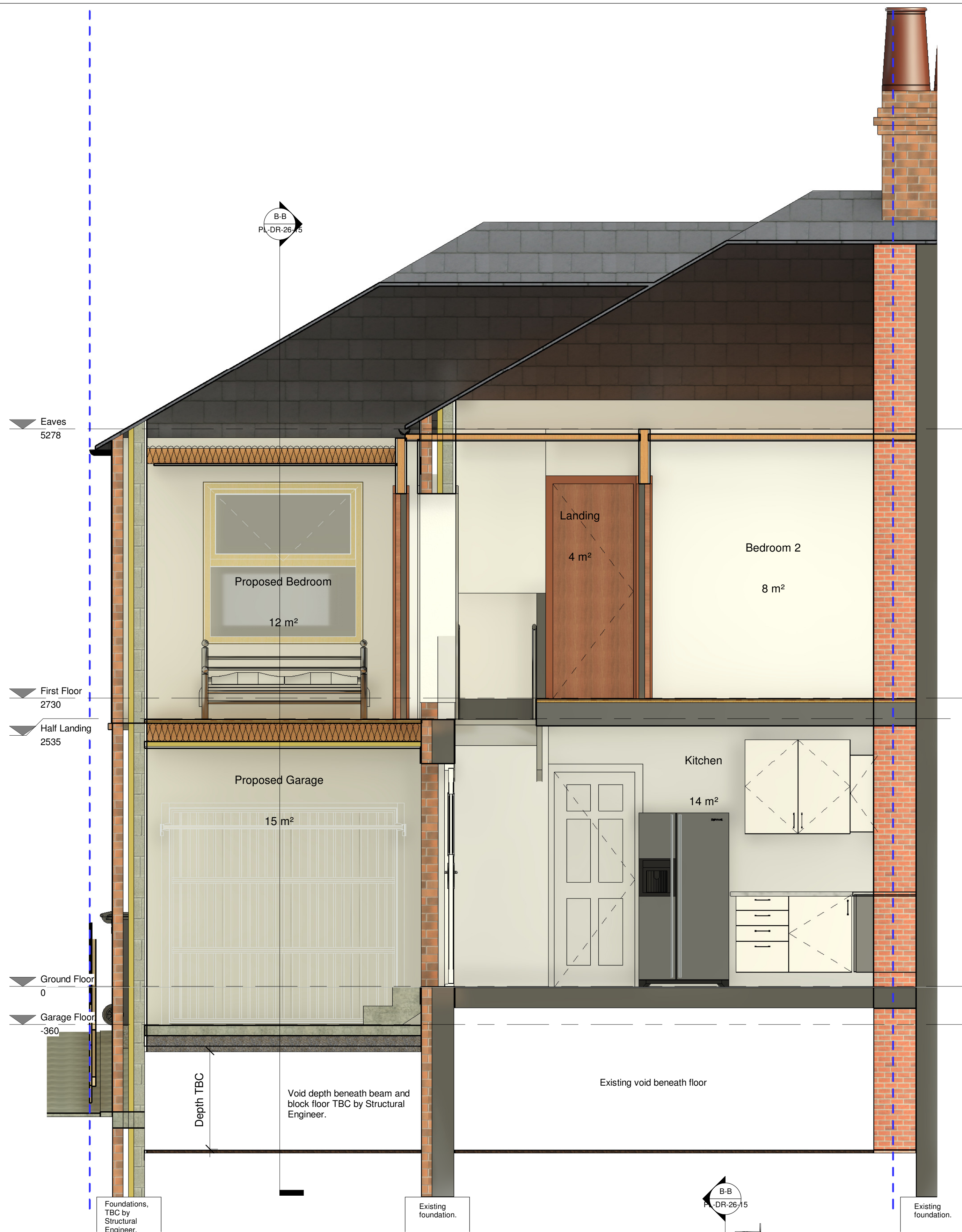
Section A-A 1 : 25
