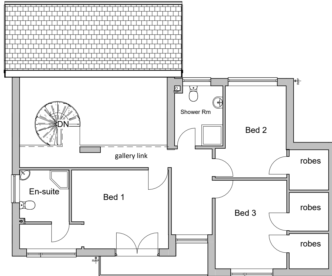
2 03a FF Existing 1 : 100
