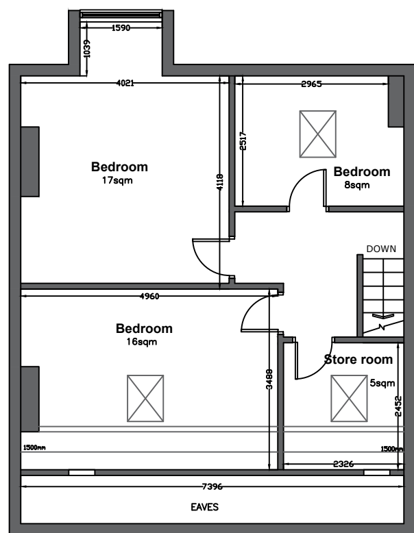
LOFT
