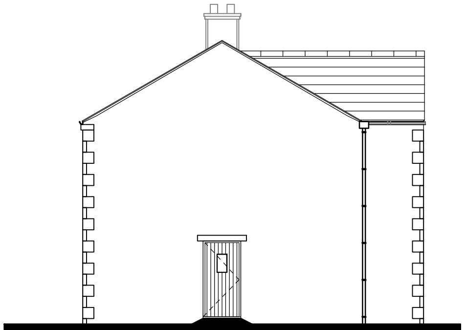
R.H. Side elevation 1:100
