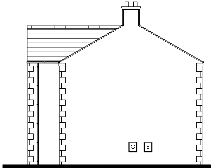
L.H. Side elevation 1:100
