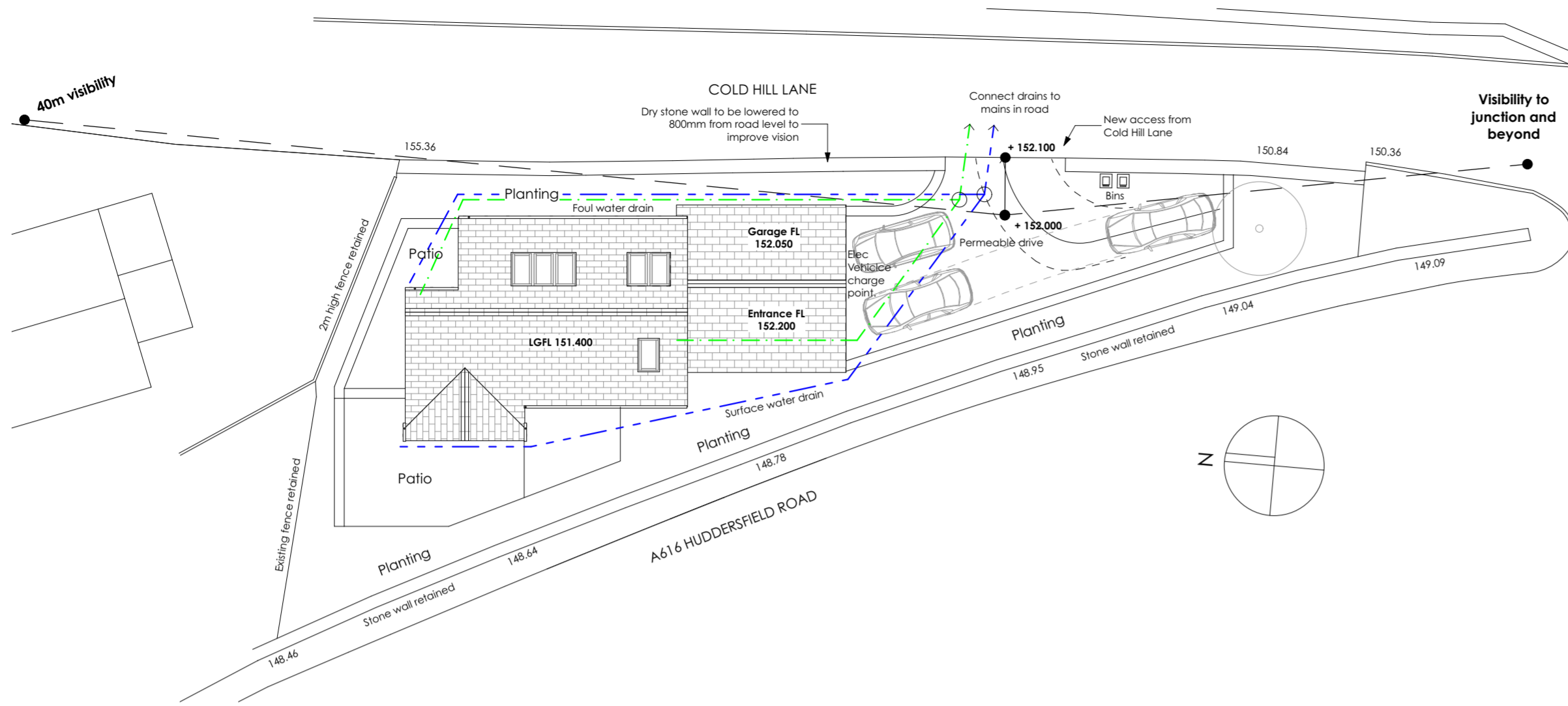
Site Plan 1:200
