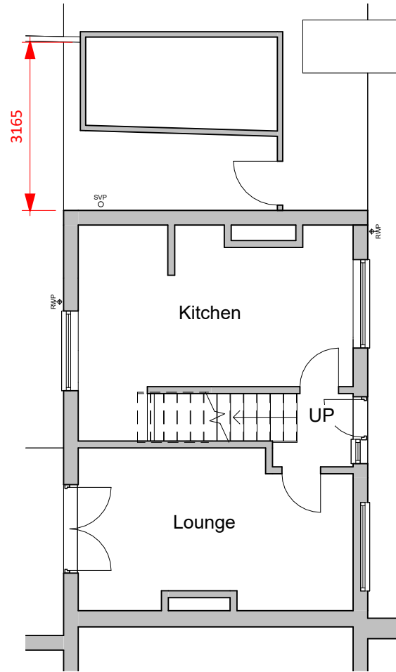
1 02a GF Existing 1 : 100
