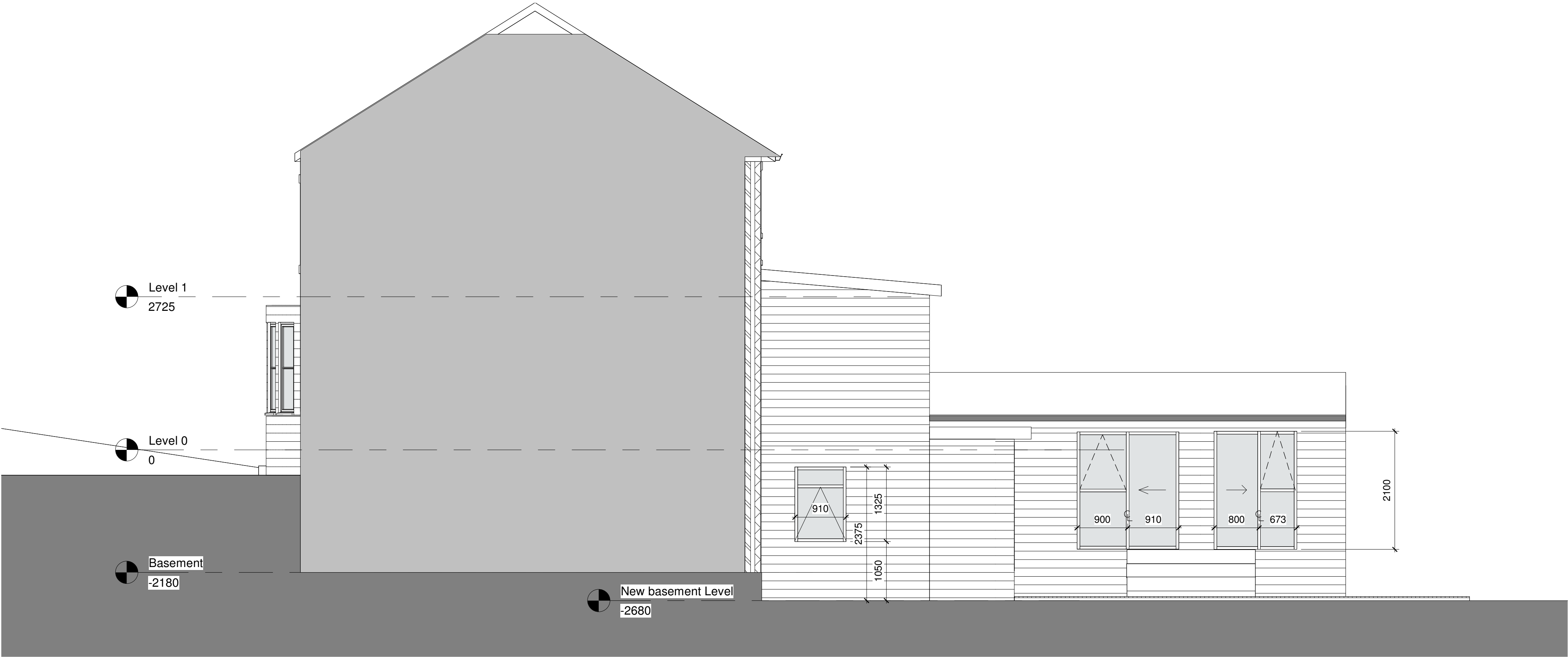
1 Section 3 1 : 50
