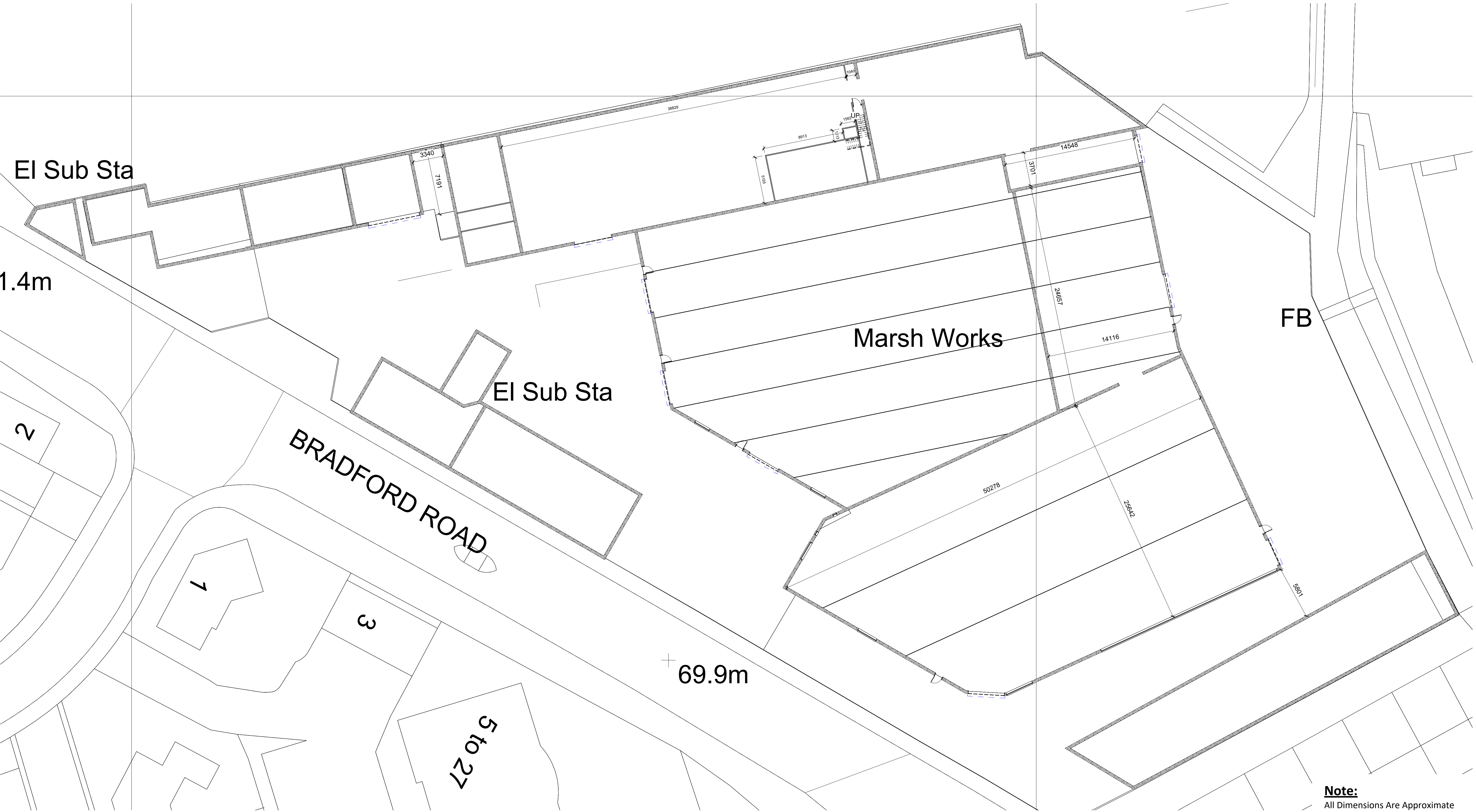
Existing Layout 1 : 200
