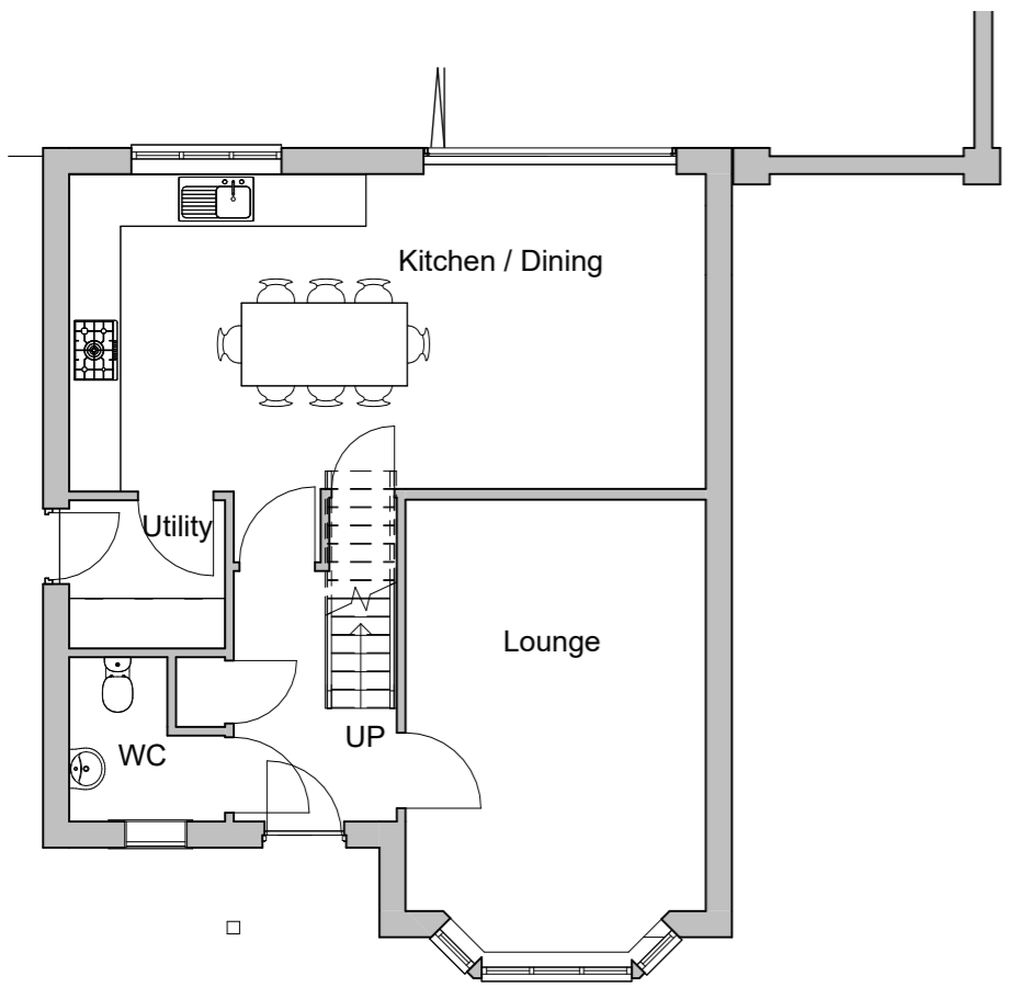
1 02a GF Existing 1 : 100
