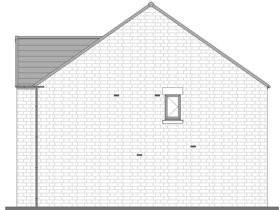
Right Elevation
