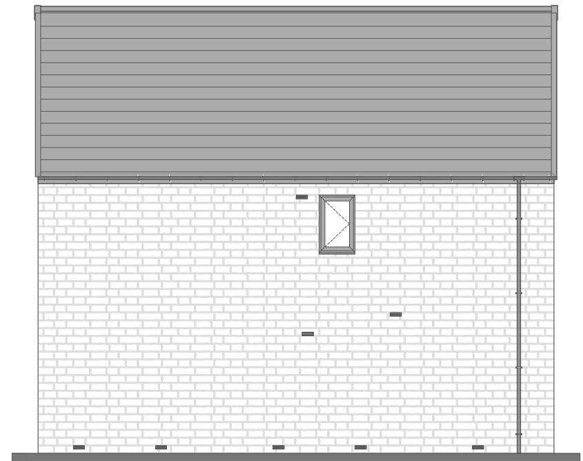
Right Elevation
