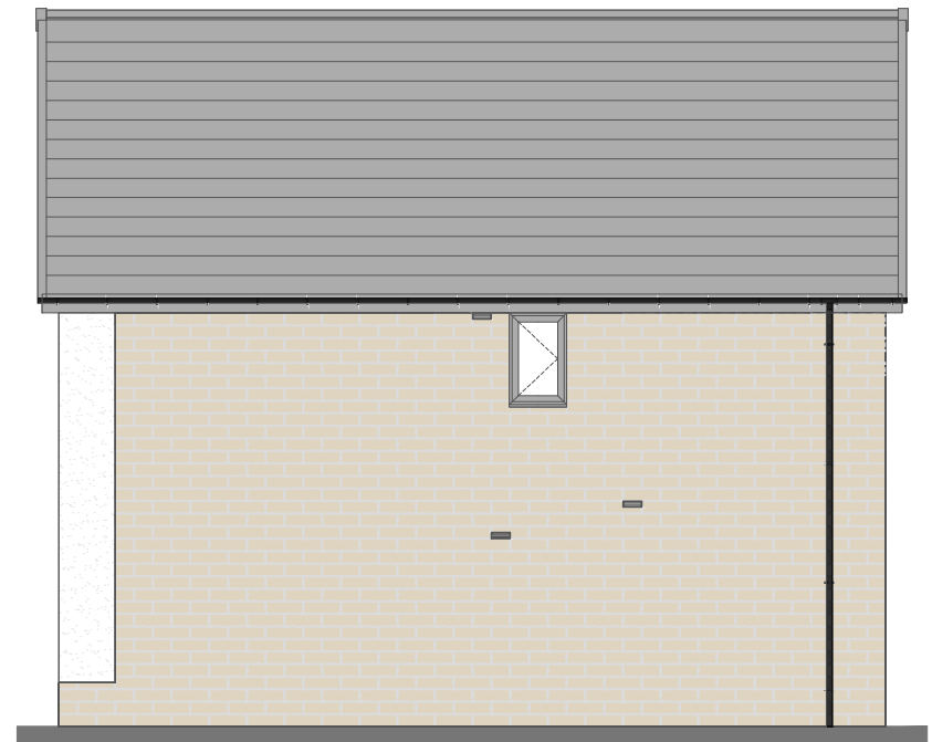
Right Elevation
