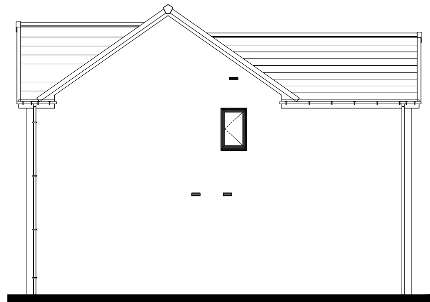
Right Elevation
