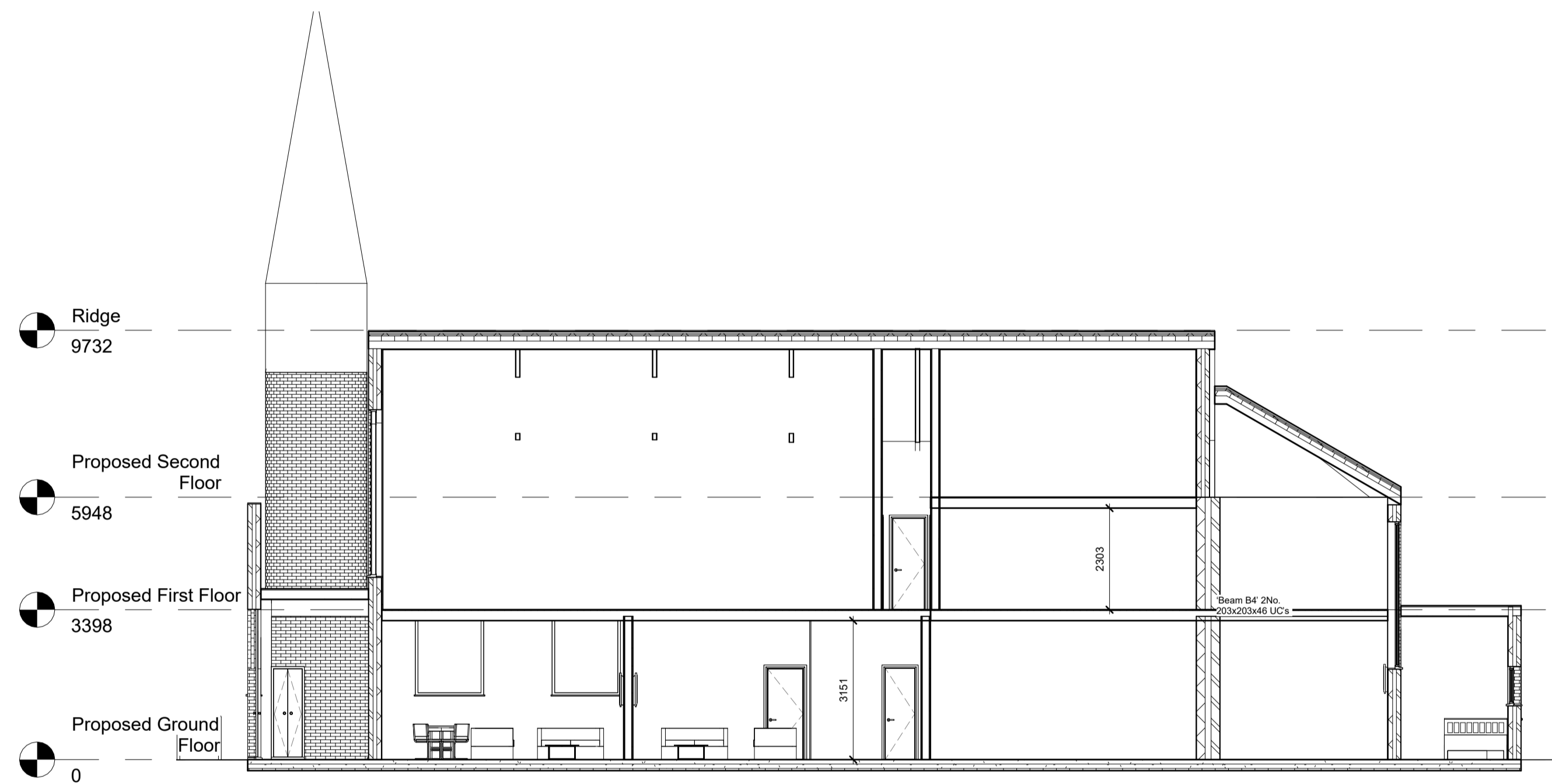
Section BB 1 : 100
