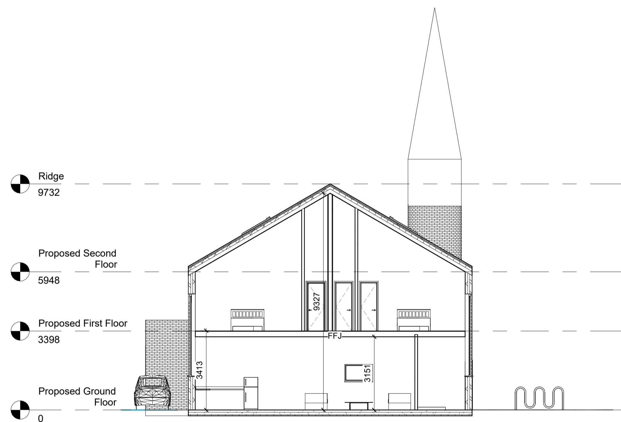
Section AA 1 : 100
