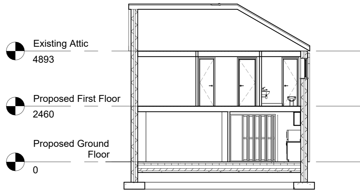
Section BB 1 : 100
