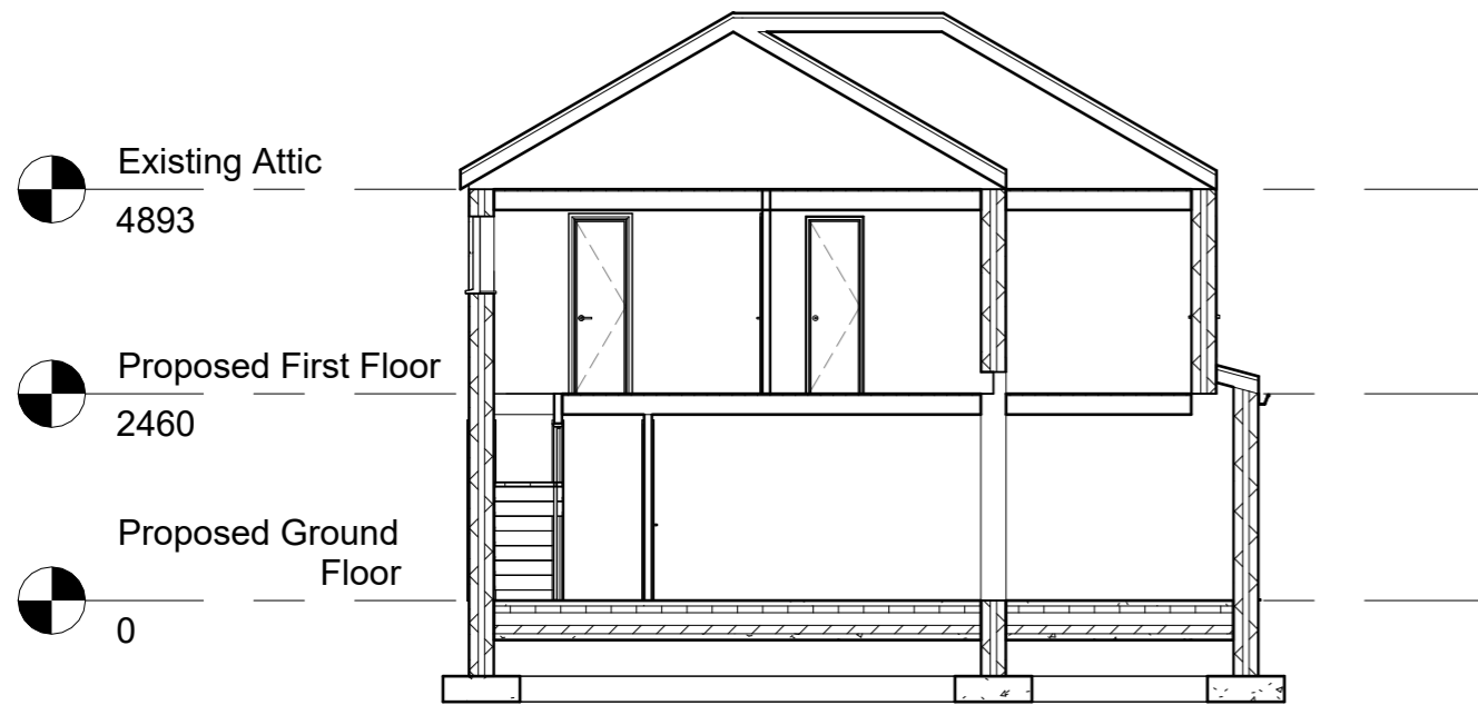
Section AA 1 : 100
