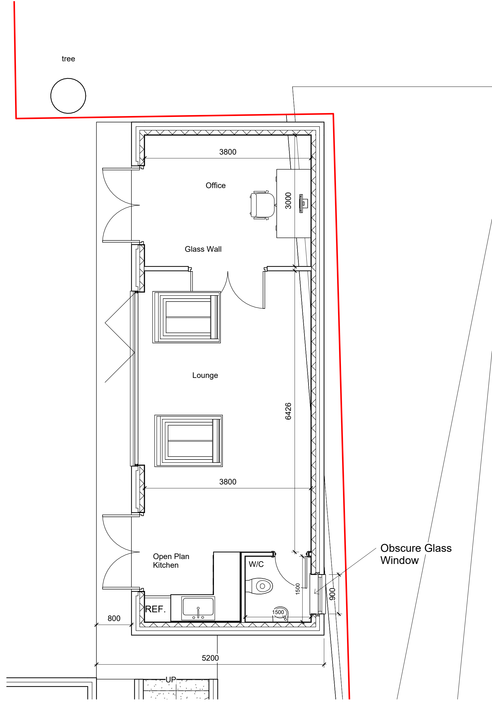
Annotation Plan 1 : 50
