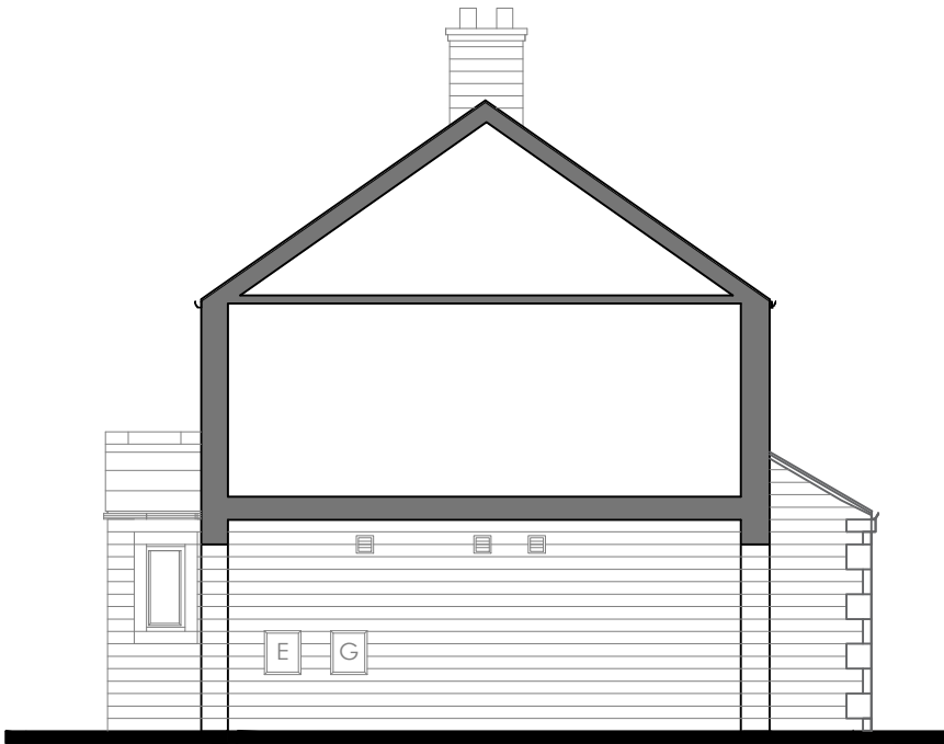
R.H. SIDE ELEVATION
