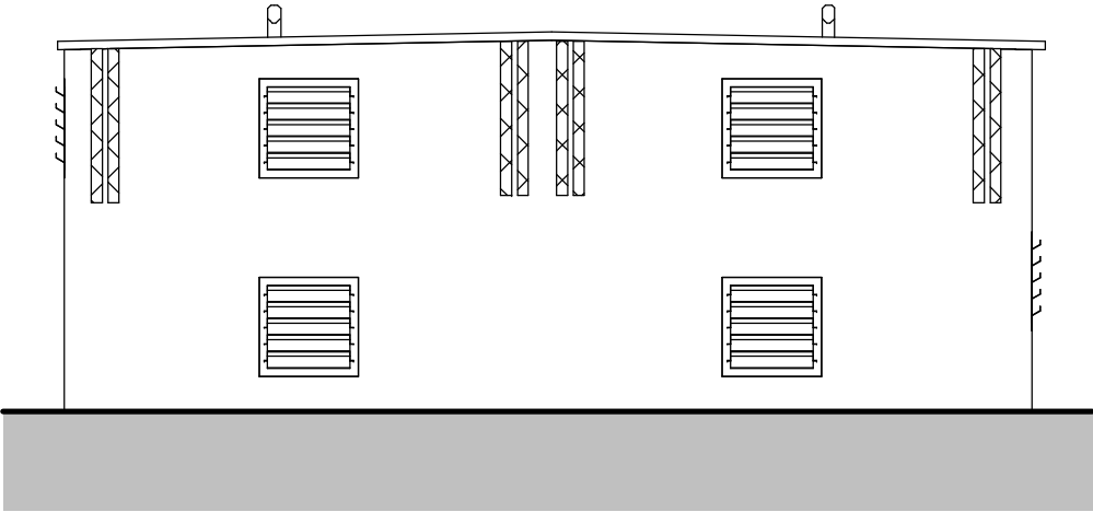
North 1 : 50
