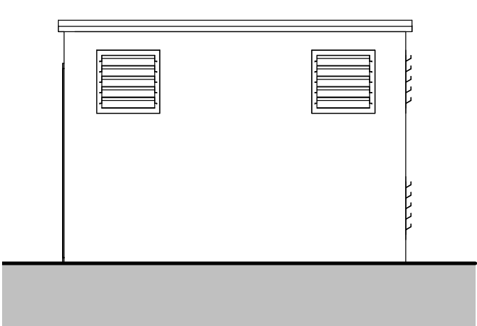
East 1 : 50
