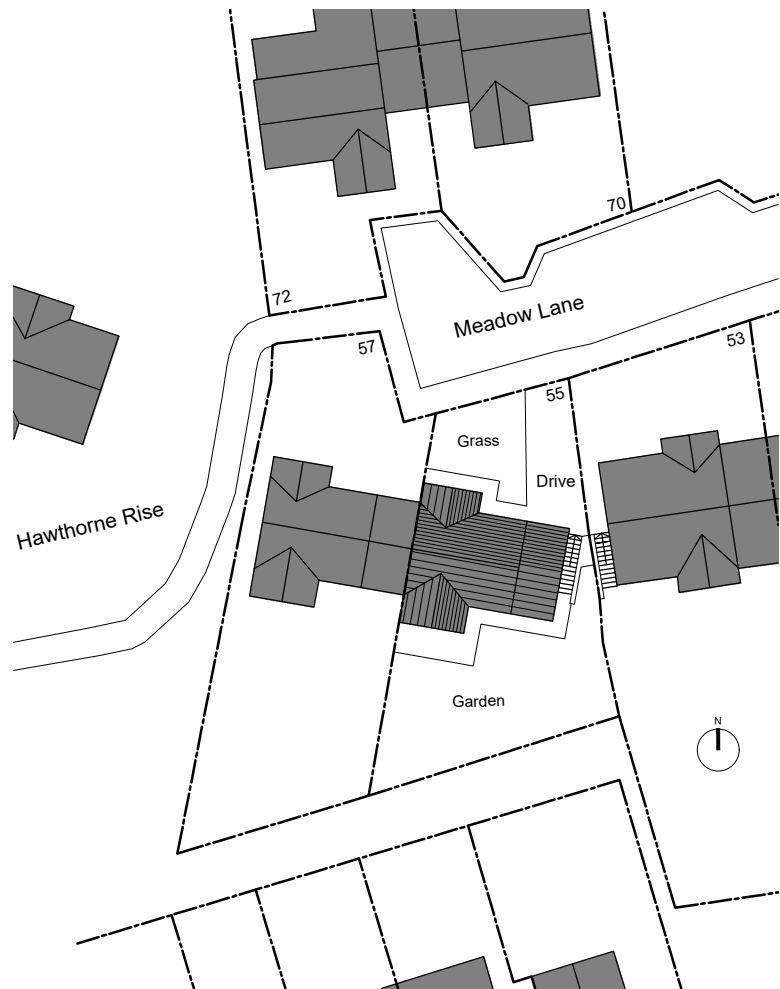
Site Plan 1:500
