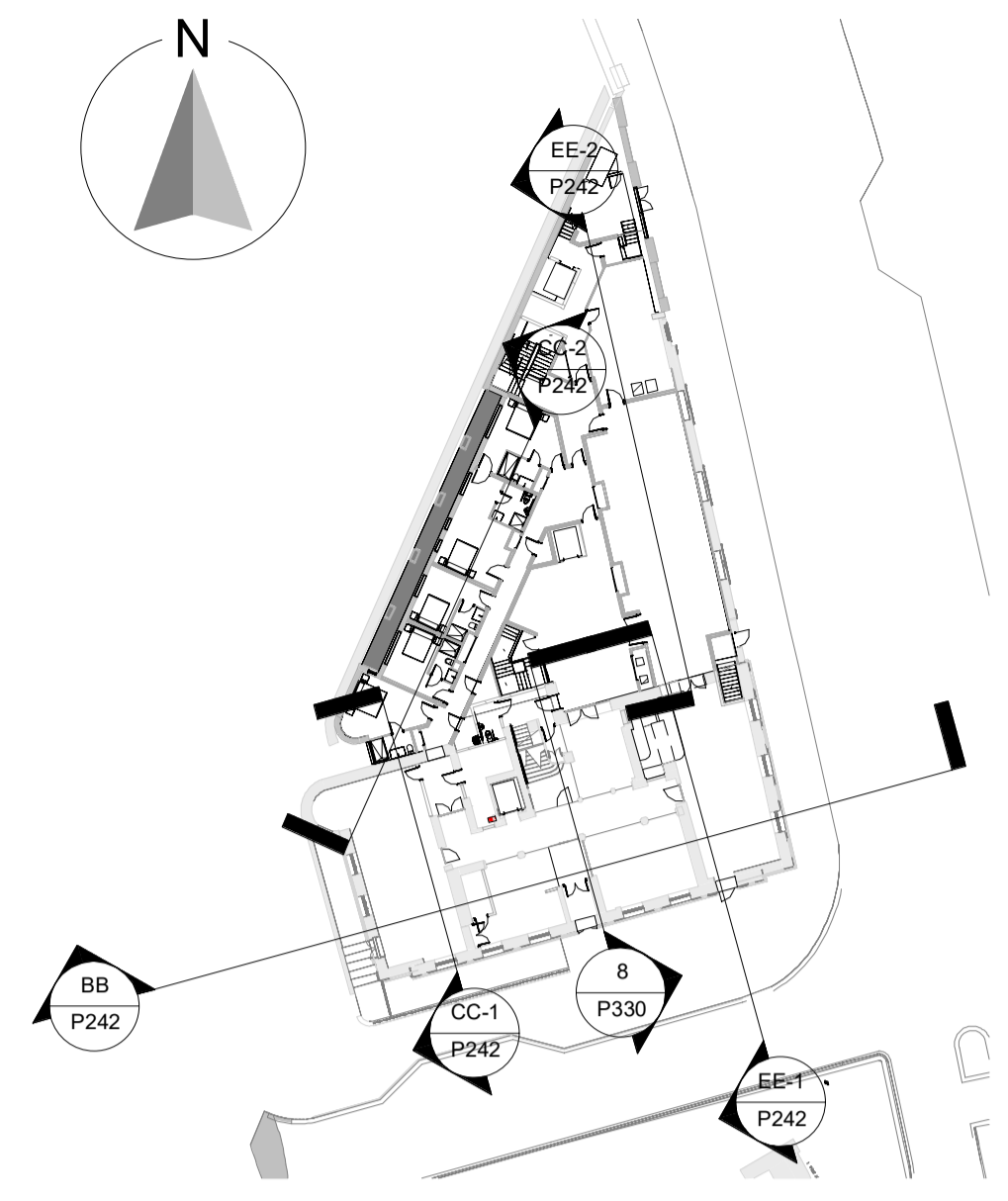
0142 Site Section Key 1 : 500
