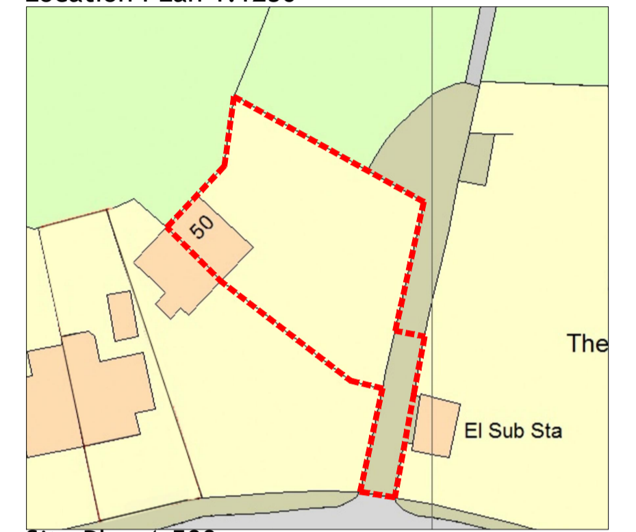
Site Plan 1:500
