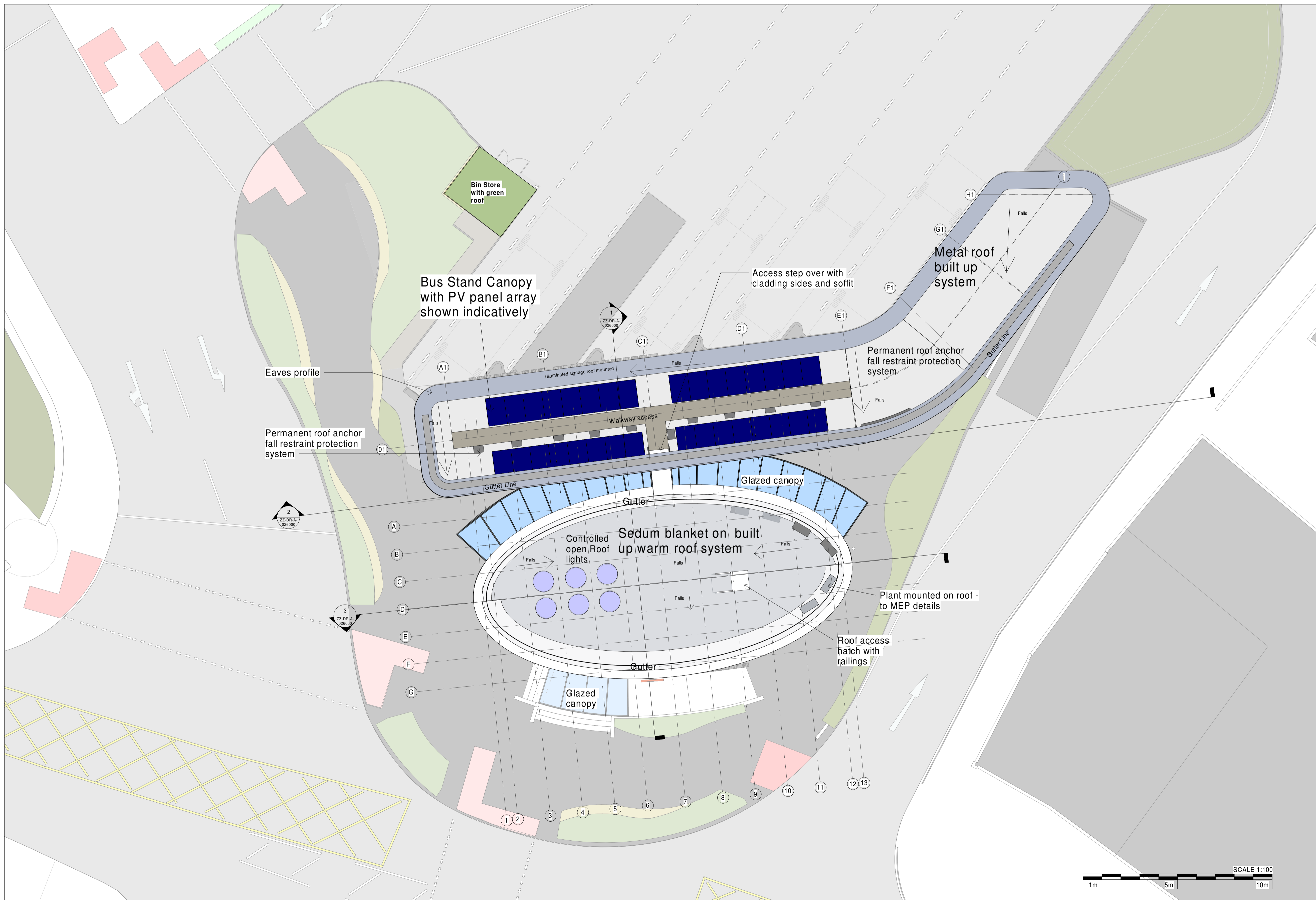
1 Roof Plan 1 : 100
