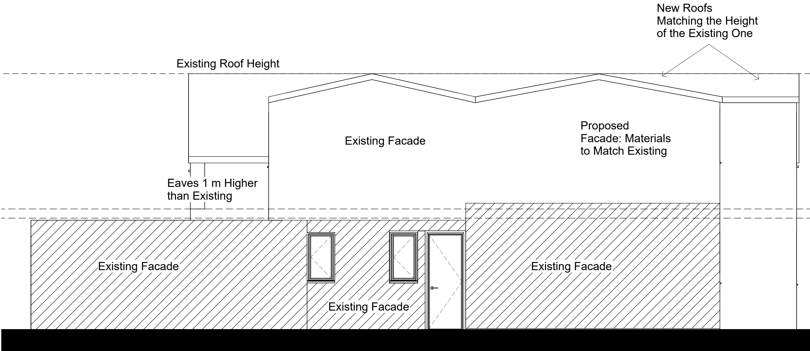
Right 1 : 50
