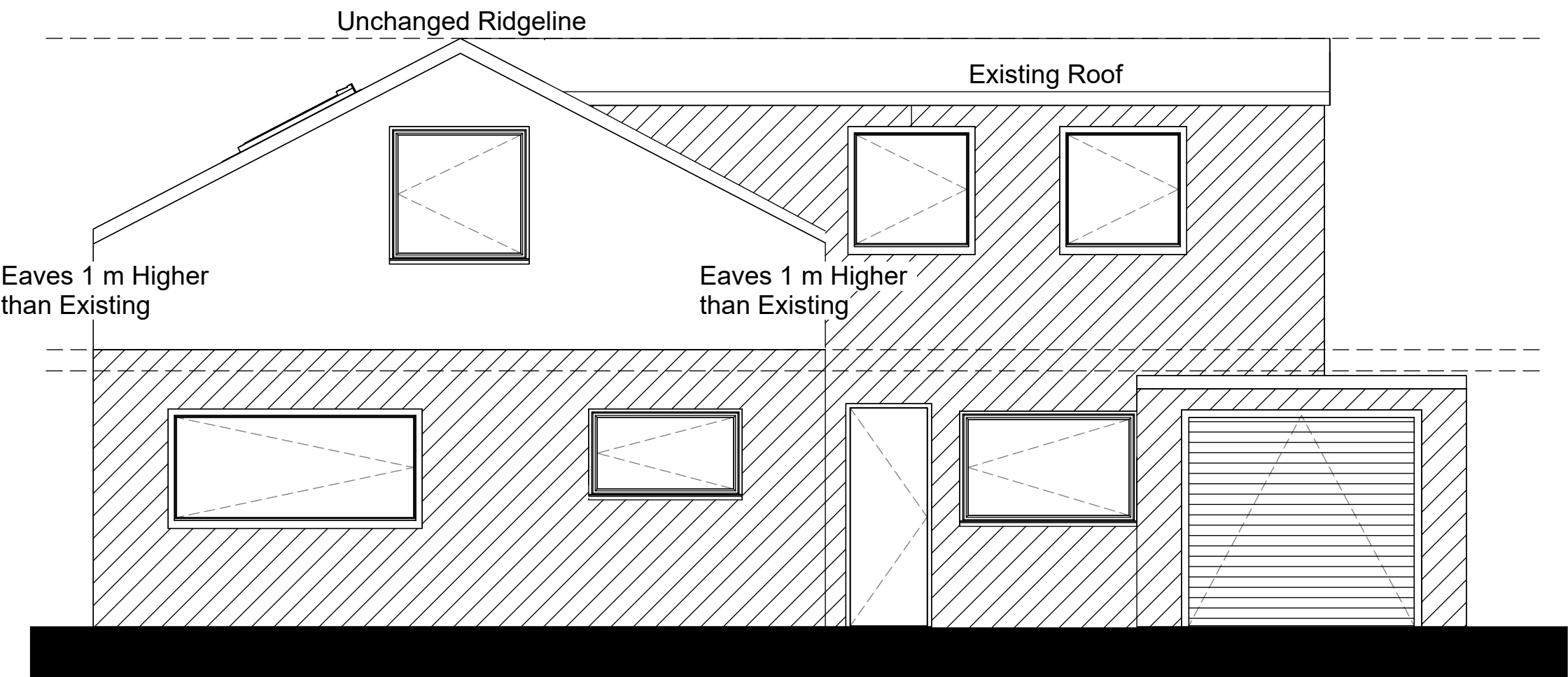
Front 1 : 50
