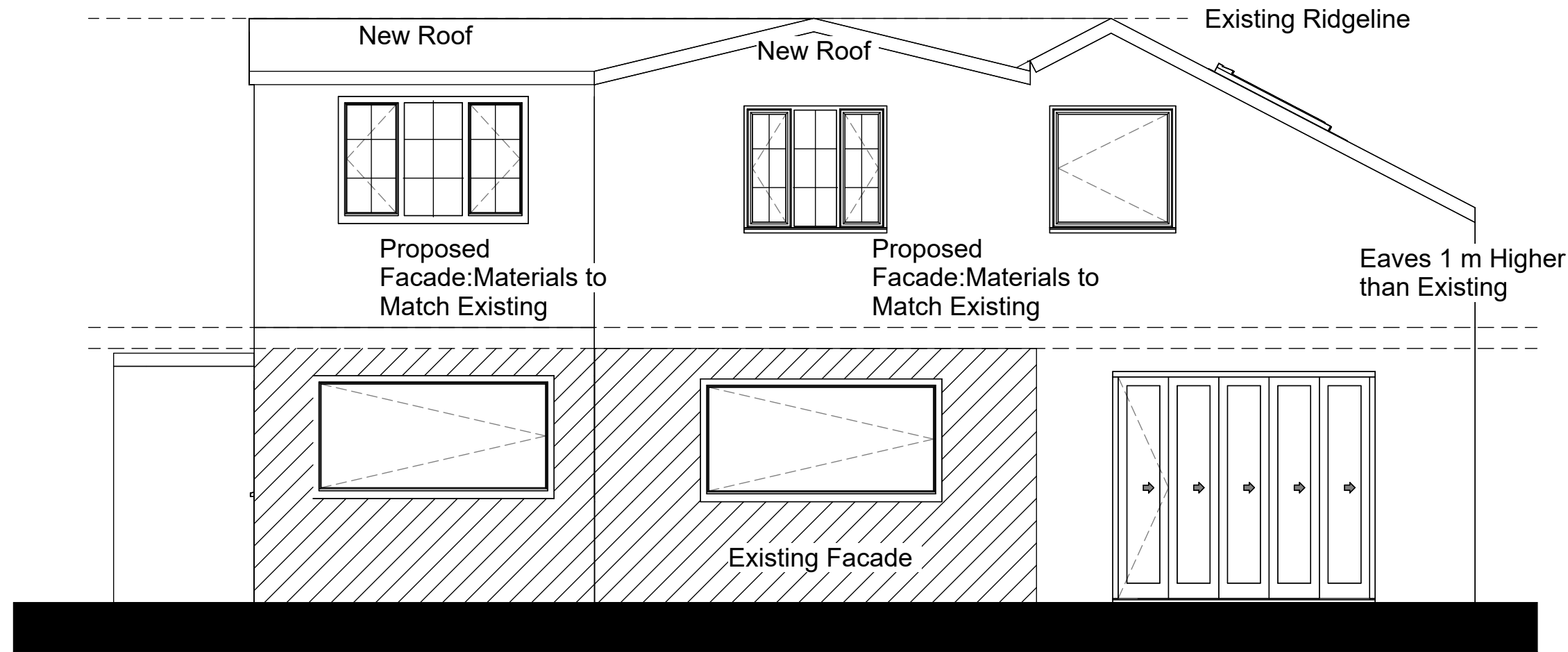
Rear 1 : 50
