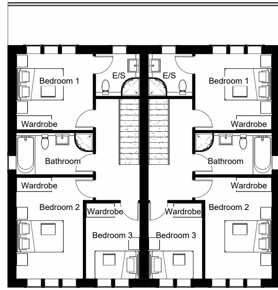
2 FFFL 1 : 100
