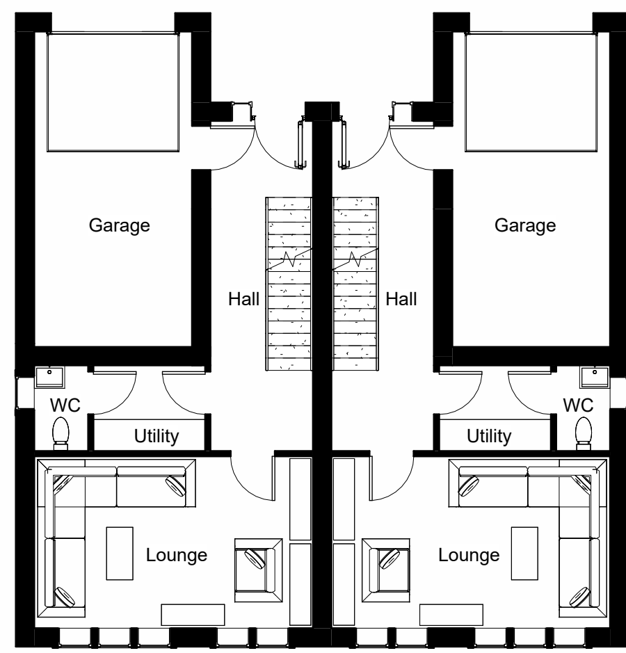
3 GFFL 1 : 100
