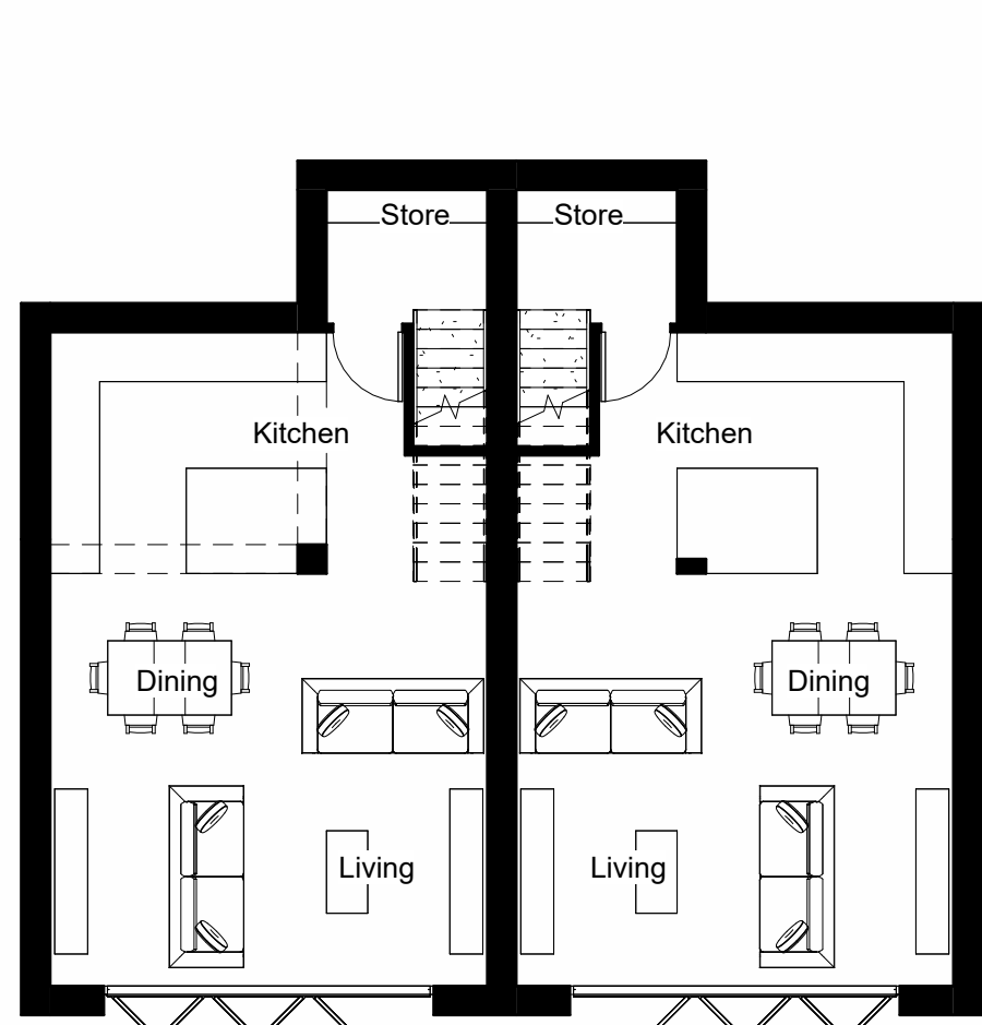
1 BFFL 1 : 100
